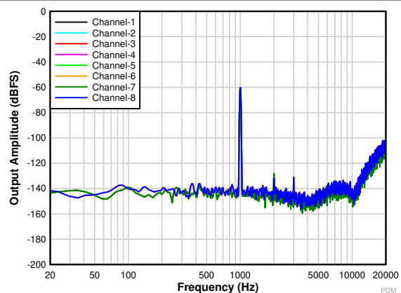
图 5-16. 输入为 -60dB r 时的 FFT
