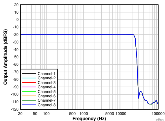
图 5-11. 输入为 -20dB 时的频率响应
