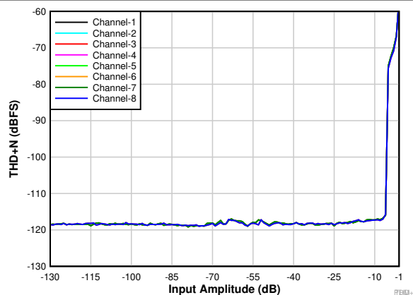
图 5-9. THD+N 与输入幅度间的关系
