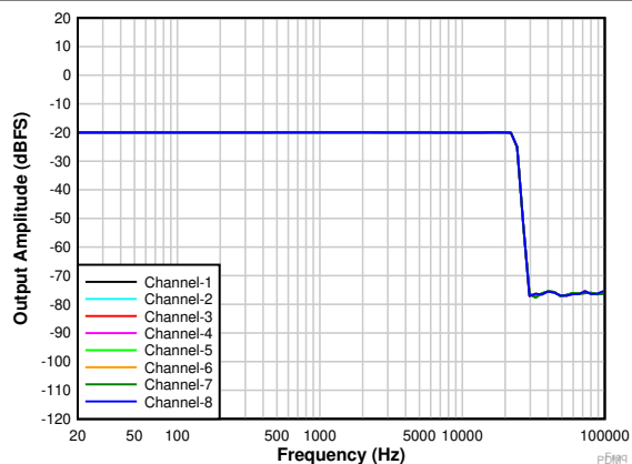
图 5-15. 输入为 -20dB r 时的频率响应
