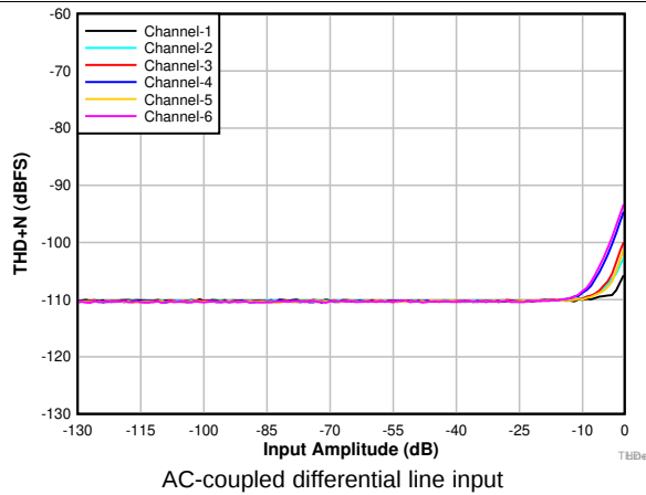
图 4. THD+N vs Input Amplitude
