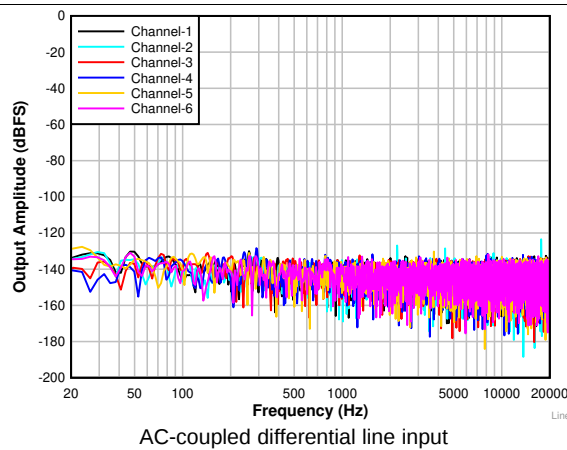
图 8. FFT With Idle Input
