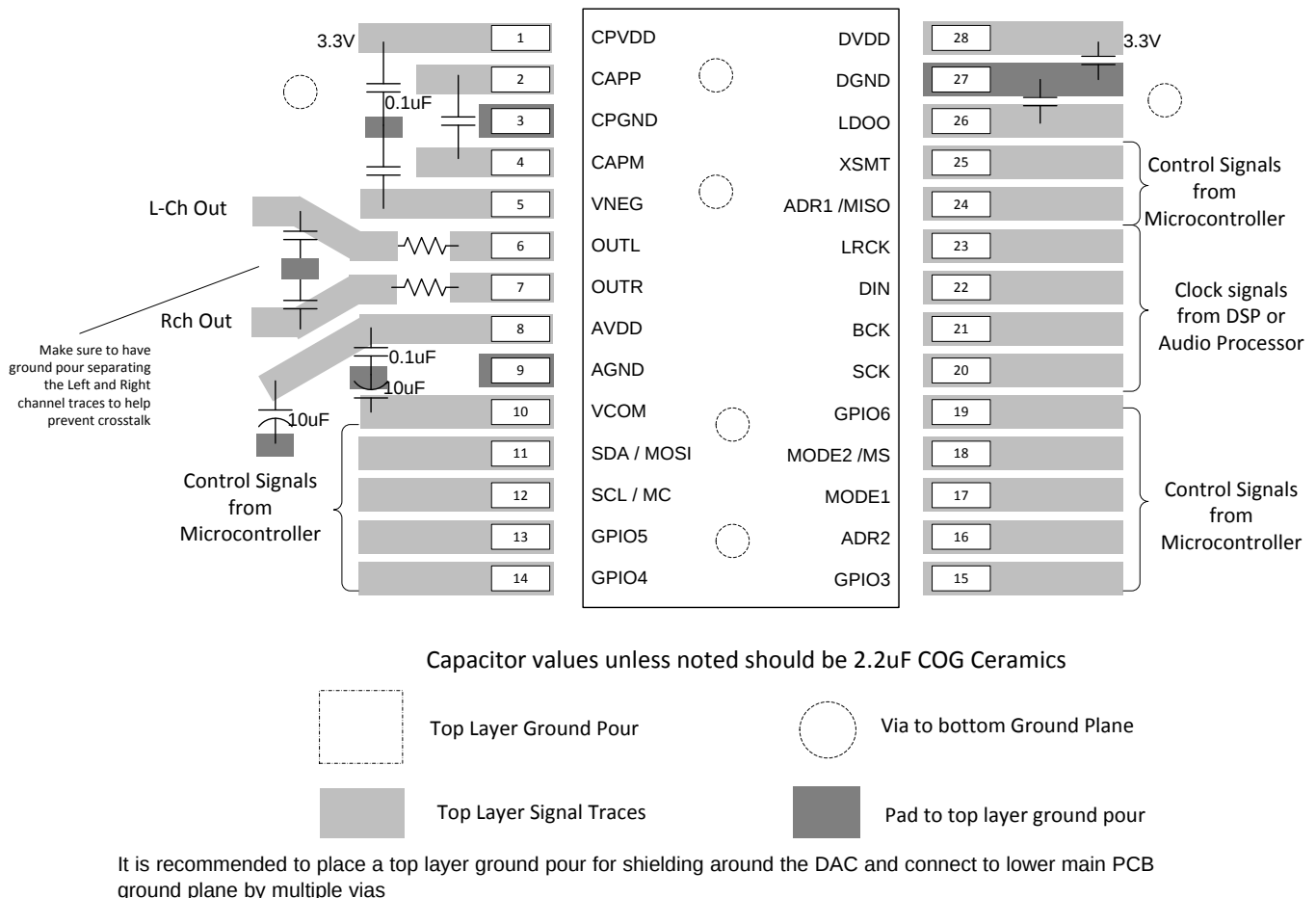
图 87. PCM514x Layout Example
