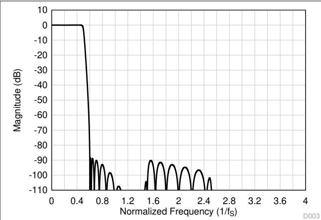
图 7-53. 超低延迟抽取滤波器幅度响应
