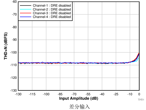
图 6-6. THD+N 与输入幅度间的关系 (DRE 已禁用)
