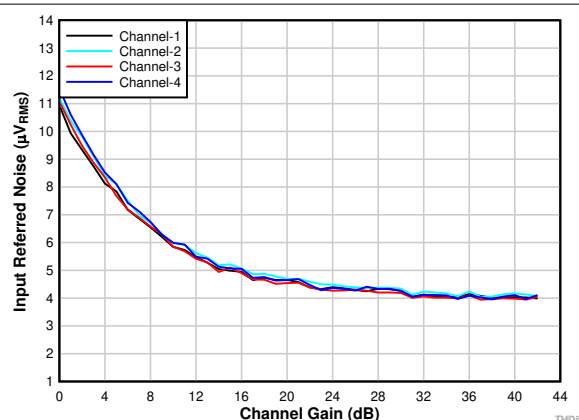
图 6-14. 以输入为基准的噪声与通道增益间的关系 单端输入
