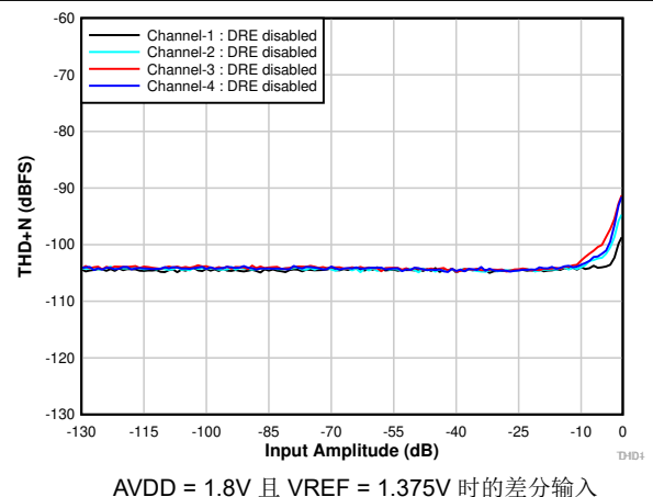
图 6-10. THD+N 与输入幅度间的关系 (DRE 已禁用)
