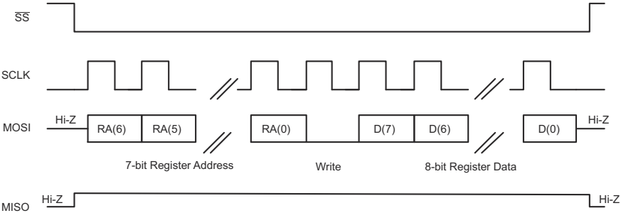
图 7-71. SPI 单字节写入传输
