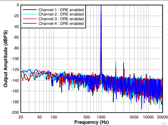
图 6-21. 输入为 -1dB 时的 FFT ( DRE 已启用 )
