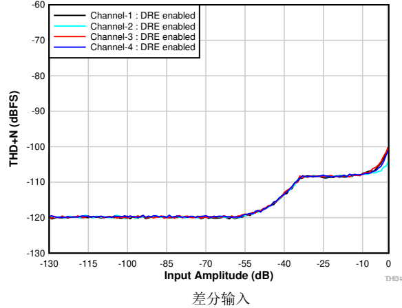
图 6-5. THD+N 与输入幅度间的关系 (DRE 已启用)
