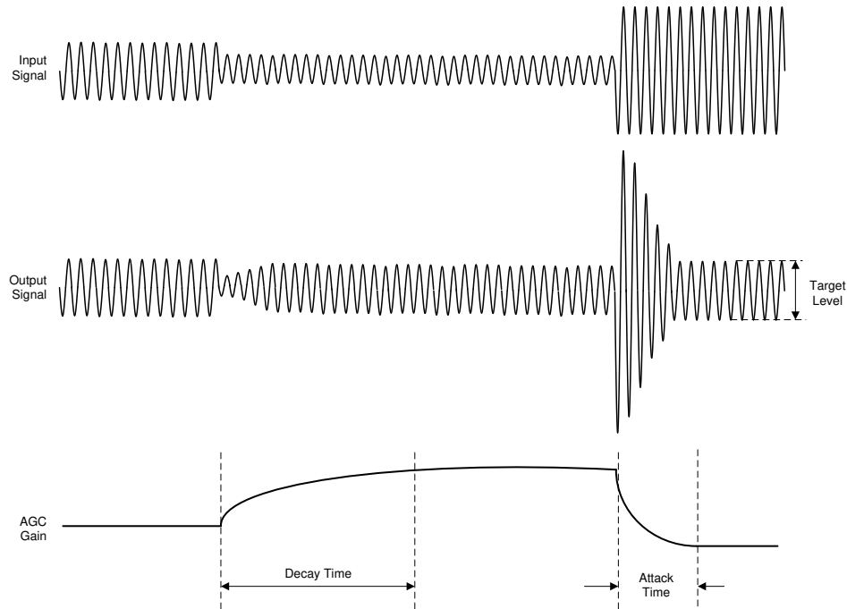
图 7-63. AGC 特性
