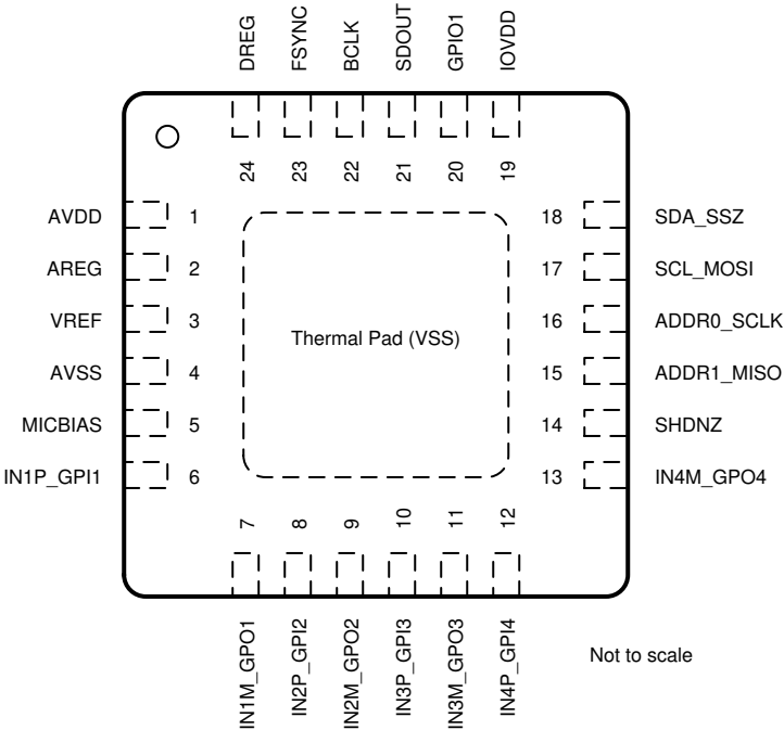
图 5-1. RTW 封装 24 引脚 WQFN (带有外露散热焊盘) 俯视图
