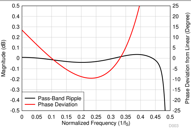
图 7-54. 超低延迟抽取滤波器通带纹波和相位偏差
