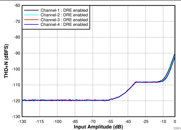
图 8-3. THD+N 与输入幅度间的关系 (DRE 已启用)
