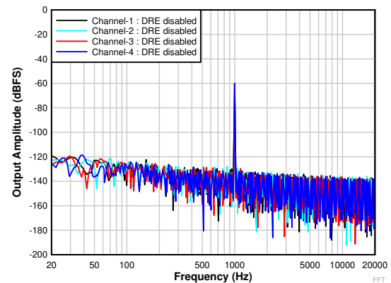
图 6-20. 具有 -60dB 输入的 FFT ( DRE 已禁用 )
