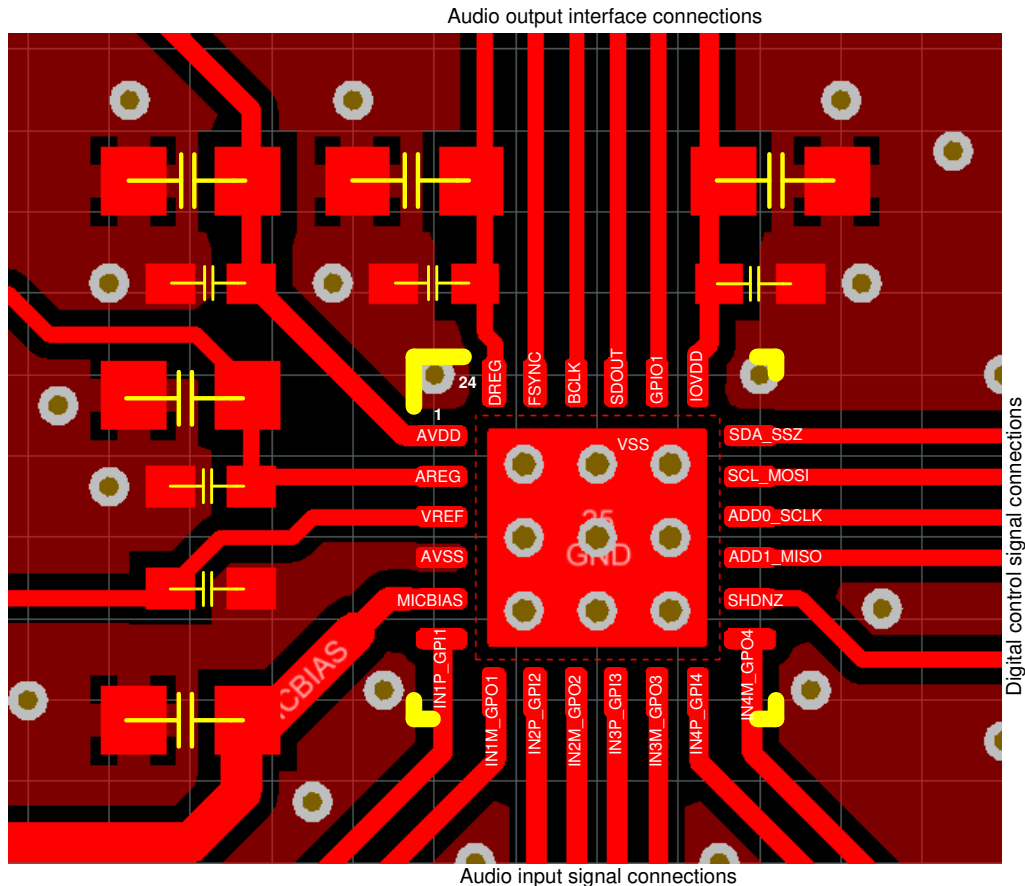
图 10-1. 布局示例
