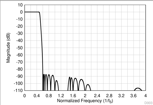
图 7-51. 超低延迟抽取滤波器幅度响应
