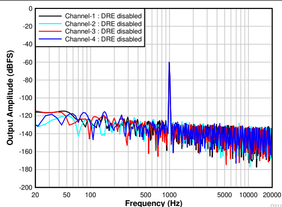
图 8-4. 具有 -60dB r 输入的 FFT (DRE 已禁用)
