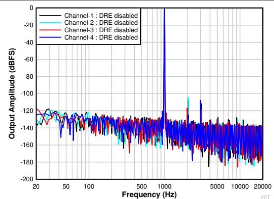
图 6-22. 具有 -1dB 输入的 FFT ( DRE 已禁用 )
