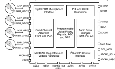
简化版方框图
