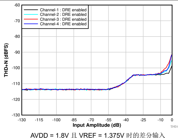
图 6-9. THD+N 与输入幅度间的关系 (DRE 已启用)
