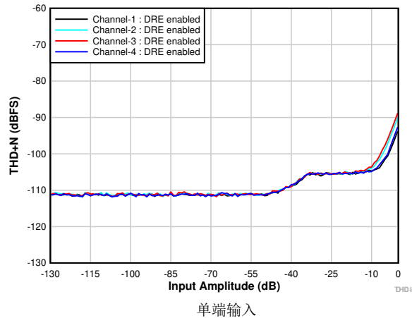
图 6-7. THD+N 与输入幅度间的关系 (DRE 已启用)
