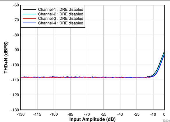
图 8-5. THD+N 与输入幅度间的关系 (DRE 已禁用)
