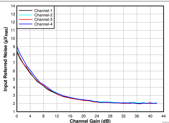
图 6-13. 以输入为基准的噪声与通道增益间的关系 差分输入
