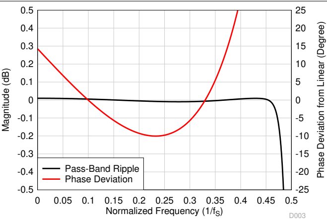
图 7-52. 超低延迟抽取滤波器通带纹波和相位偏差
