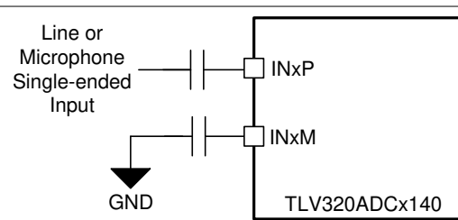
图 7-15. 单端交流耦合输入连接
