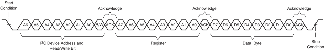
图 7-67. I 2 C 单字节写入传输
