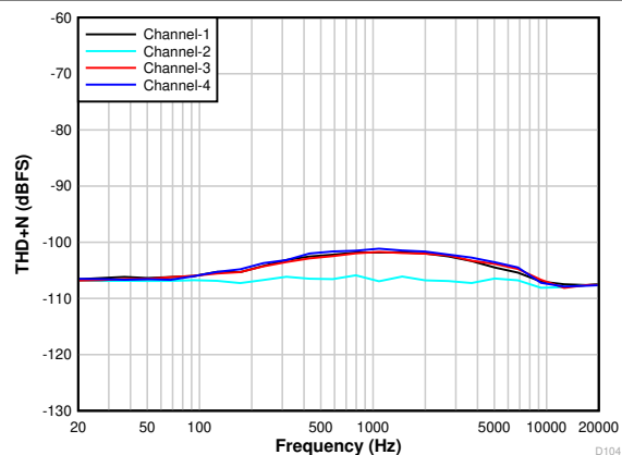
图 6-12. 输入为 -1dBm 时 THD+N 与输入频率间的关系
