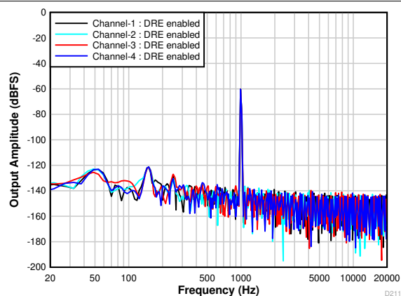
图 8-2. 具有 -60dB r 输入的 FFT (DRE 已启用)
