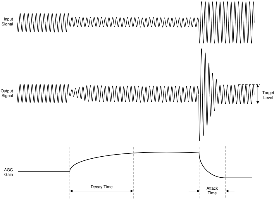
图 7-63. AGC 特性
