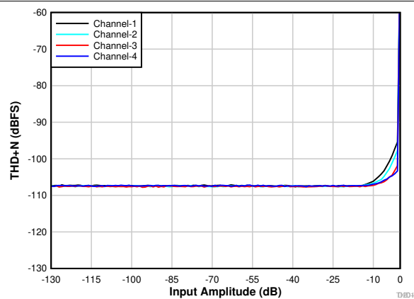
图 9-3. THD+N 与输入幅度间的关系
