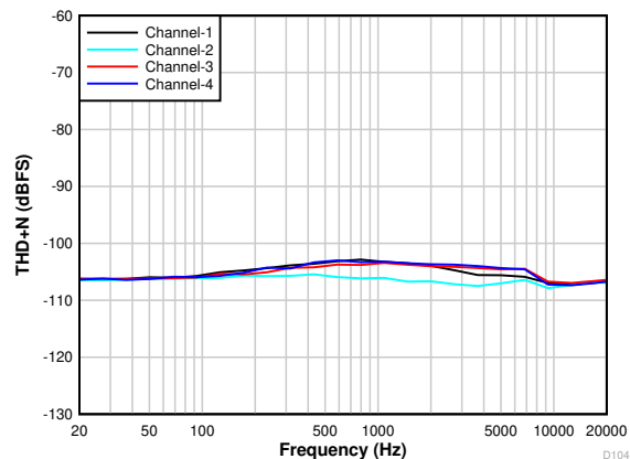
图 6-9. 输入为 -1dBm 时 THD+N 与输入频率间的关系
