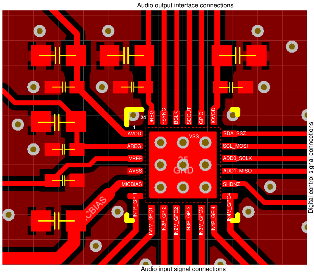
图 9-6. 布局示例
