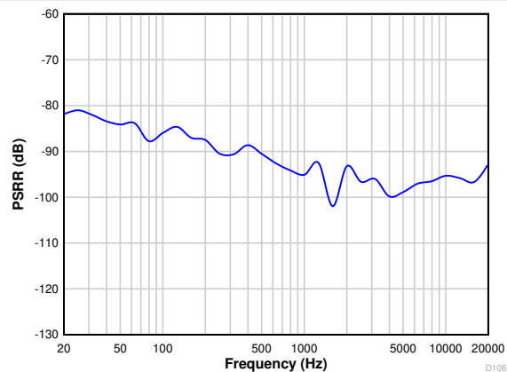
图 6-13. 100mV pp 振幅下电源抑制比与纹波频率间的关系
