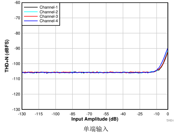
图 6-6. THD+N 与输入幅度间的关系
