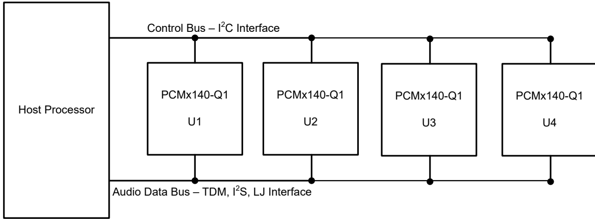
图 7-13. 多个 PCM3140-Q1 器件具有共享控制和音频数据总线
