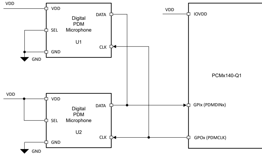
图 7-64. 数字 PDM 麦克风与 PCM3140-Q1 的连接图
