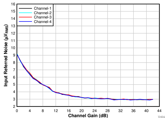
图 6-10. 以输入为基准的噪声与通道增益间的关系
