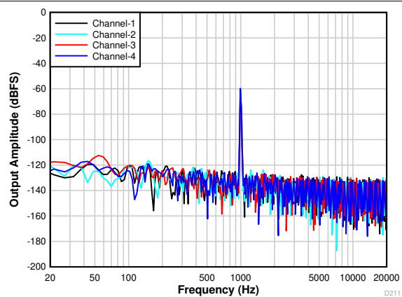
图 9-2. 具有 -60dB 输入的 FFT
