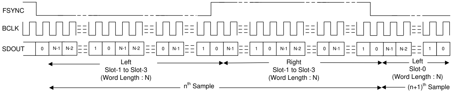
图 7-7. I²S 协议时序 (无空闲 BCLK 周期, TX_OFFSET = 0)
