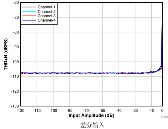
图 6-5. THD+N 与输入幅度间的关系
