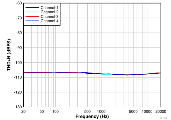
图 6-8. 输入为 -60dB 时 THD+N 与输入频率间的关系
