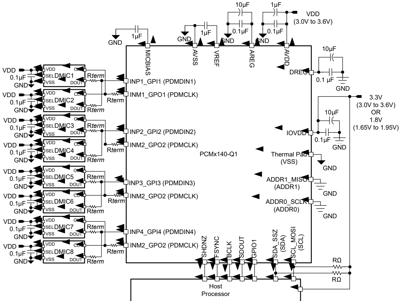
图 9-4. 八通道数字 PDM 麦克风录音图
