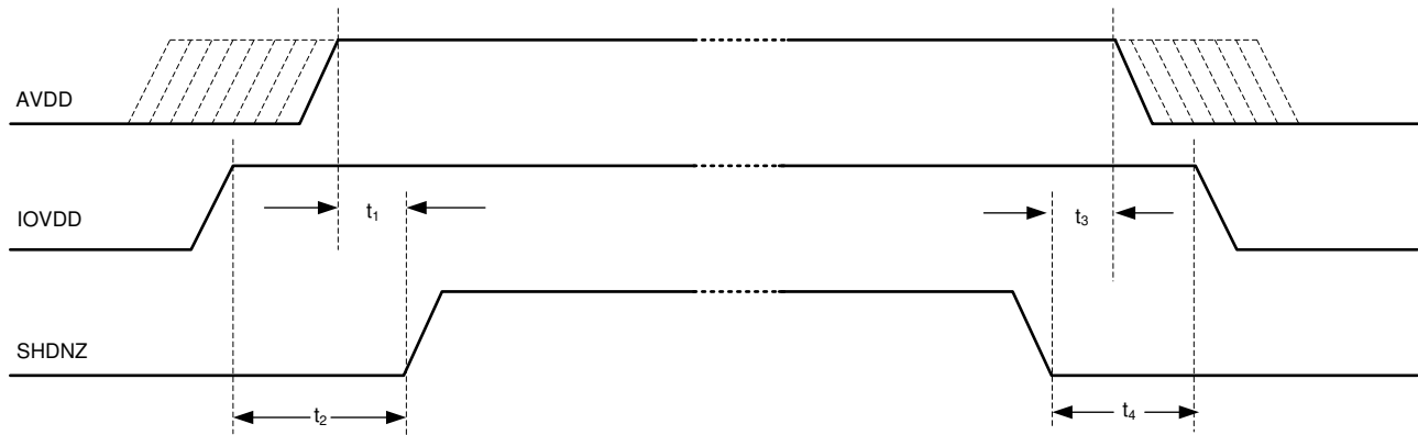
图 9-5. 电源时序要求时序图
