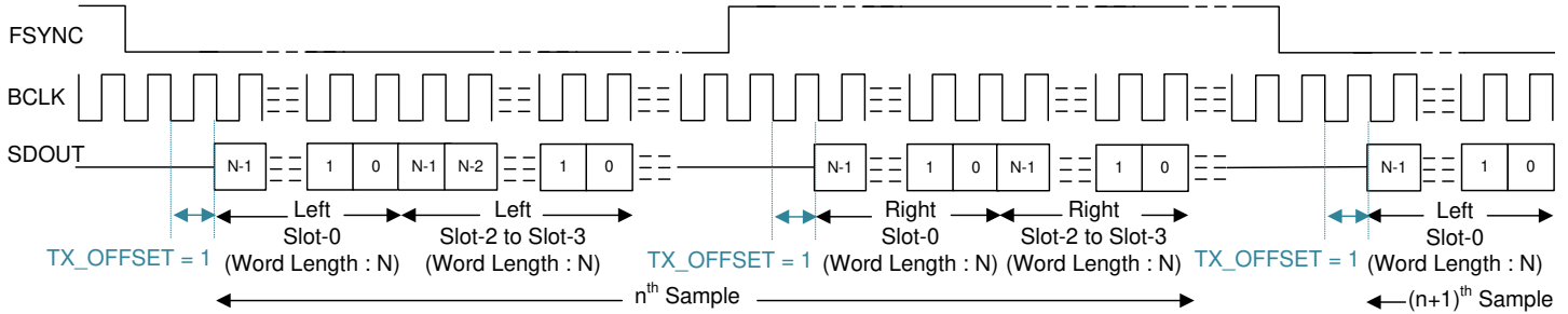
图 7-6. I²S 协议时序 (TX_OFFSET = 1)
