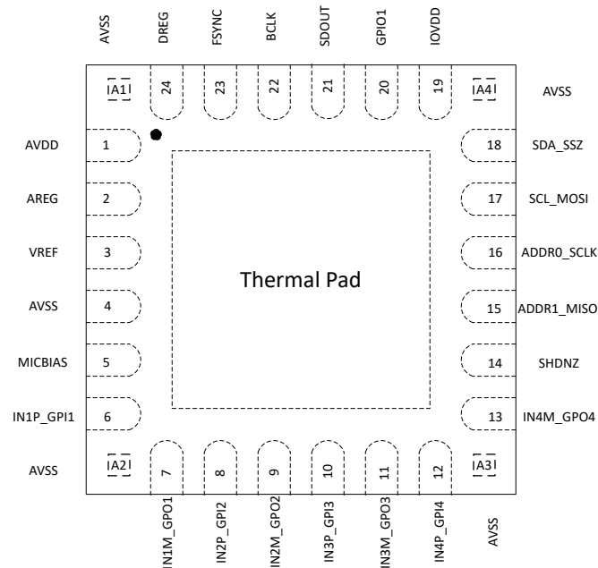
图 5-1. RGE 封装 24 引脚 VQFN (带有外露散热焊盘) 俯视图
