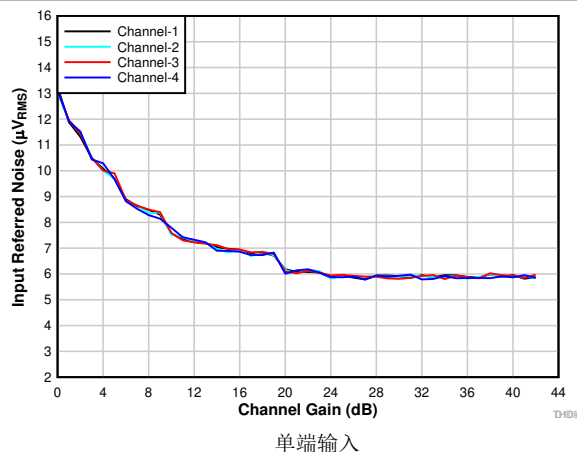
图 6-11. 以输入为基准的噪声与通道增益间的关系
