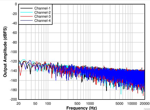
图 6-14. 空闲输入时的 FFT
