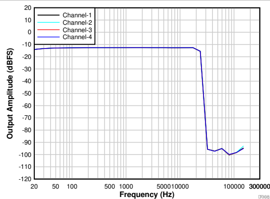
图 6-12. 输入为 -12dBm 时的频率响应
