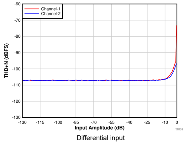
图 7-4. THD+N vs Input Amplitude
