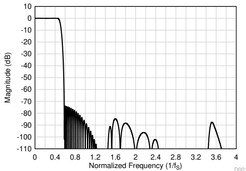
图 6-18. 线性相位抽取滤波器幅度响应
