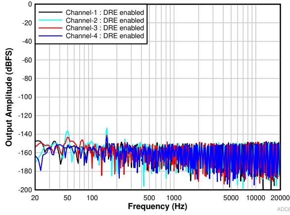
图 5-8. 空闲输入时的 FFT (DRE 已启用)
