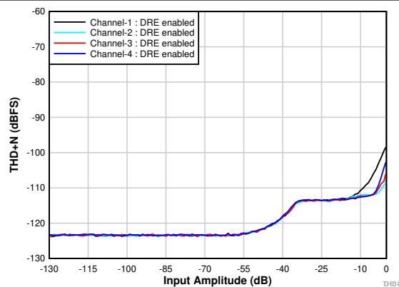
图 5-2. THD+N 与输入幅度间的关系 (DRE 已启用)
