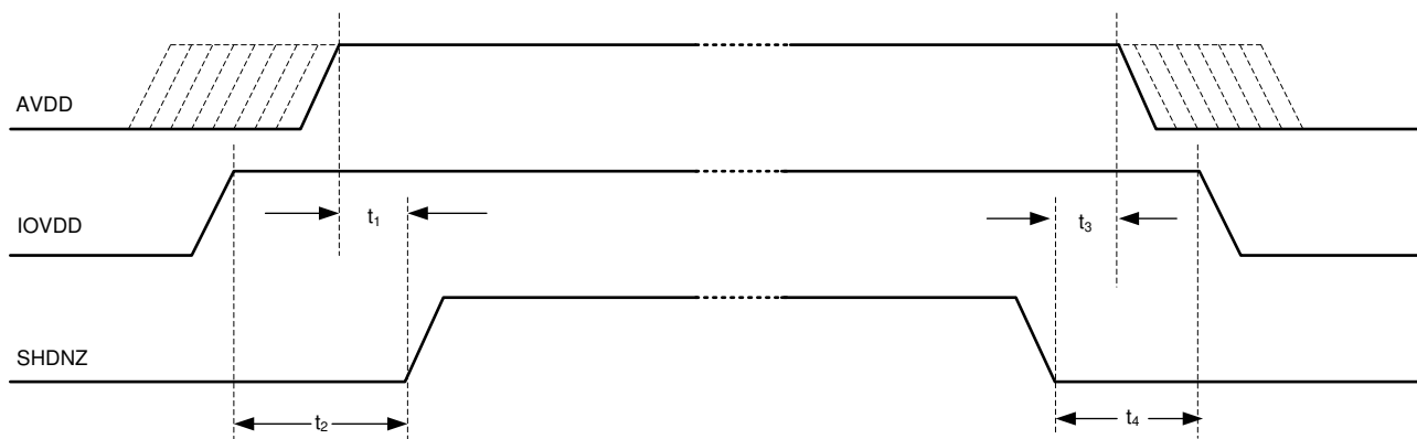
图 7-6. 电源时序要求时序图
