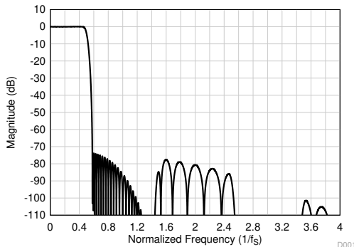
图 6-16. 线性相位抽取滤波器幅度响应
