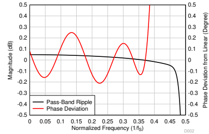
图 6-25. 低延迟抽取滤波器通带纹波和相位偏差
