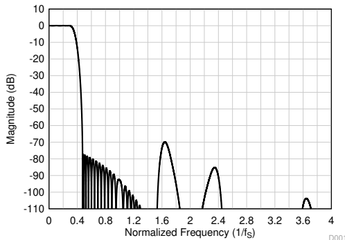
图 6-22. 线性相位抽取滤波器幅度响应
