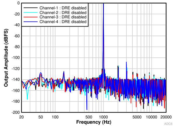
图 5-13. 具有 -1\text{dB} 输入的 FFT (DRE 已禁用)
