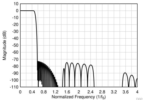
图 6-10. 线性相位抽取滤波器幅度响应
