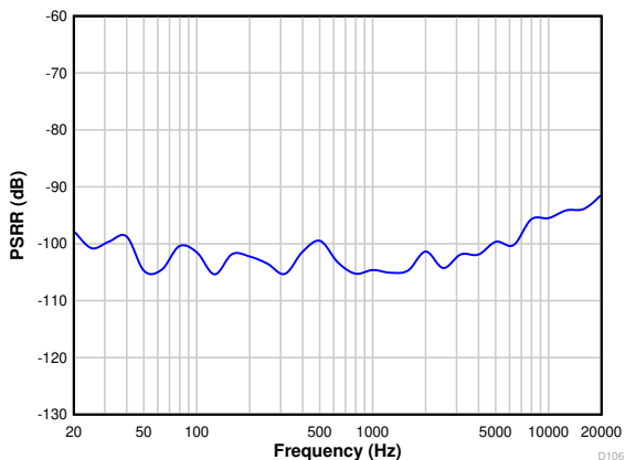
图 5-7. 100\text{mV}_{PP} 振幅下电源抑制比与纹波频率间的关系
