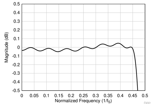
图 6-17. 线性相位抽取滤波器通带纹波
