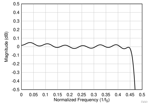
图 6-11. 线性相位抽取滤波器通带纹波
