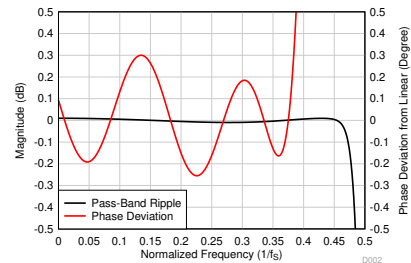
图 6-27. 低延迟抽取滤波器通带纹波和相位偏差
