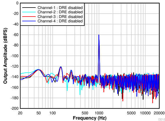
图 7-4. 具有 -60dB r 输入的 FFT (DRE 已禁用)
