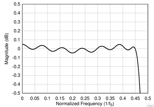
图 6-21. 线性相位抽取滤波器通带纹波
