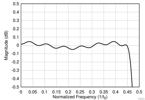
图 6-19. 线性相位抽取滤波器通带纹波
