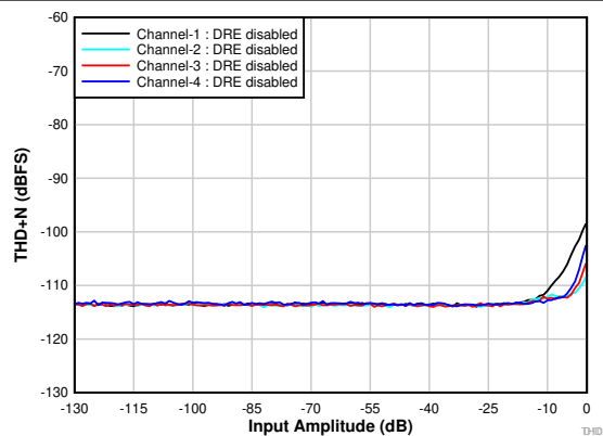
图 5-3. THD+N 与输入幅度间的关系 (DRE 已禁用)
