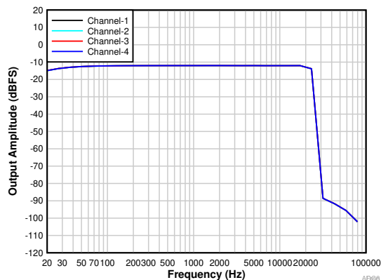
图 5-6. 频率响应 输入为 -12\text{dB}
