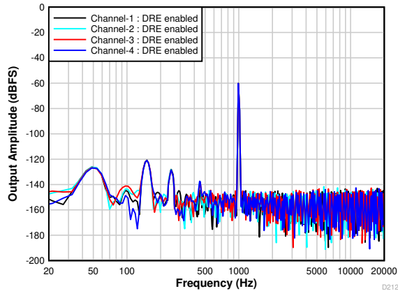
图 7-2. 具有 -60dB r 输入的 FFT (DRE 已启用)
