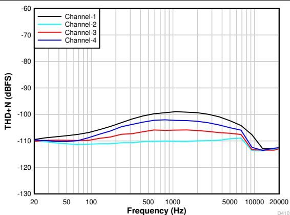
图 5-5. THD+N 与输入频率间的关系 输入为 -1\text{dB}
