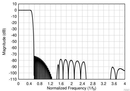
图 6-14. 线性相位抽取滤波器幅度响应
