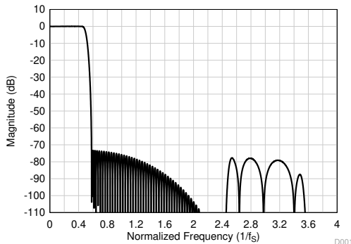
图 6-12. 线性相位抽取滤波器幅度响应
