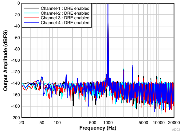
图 5-12. 具有 -1\text{dB} 输入的 FFT (DRE 已启用)
