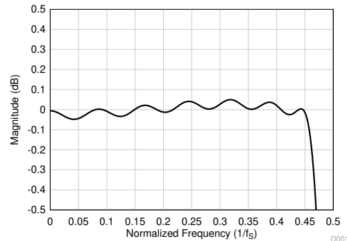
图 6-13. 线性相位抽取滤波器通带纹波
