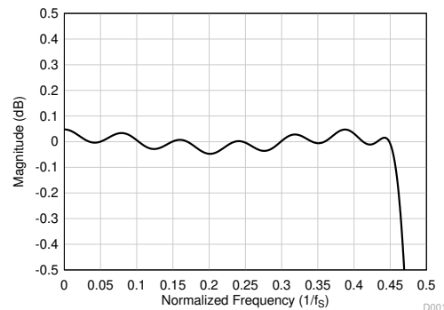
图 6-15. 线性相位抽取滤波器通带纹波
