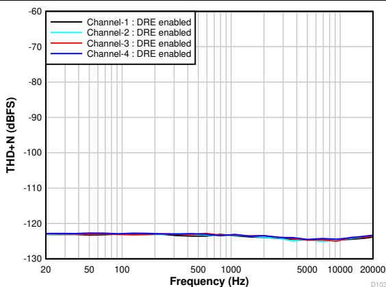
图 5-4. THD+N 与输入频率间的关系 输入为 -60\text{dB}
