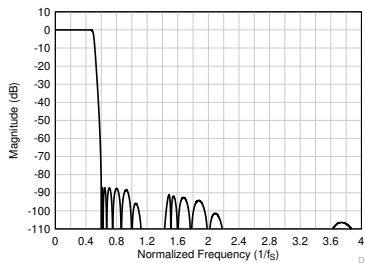
图 6-26. 低延迟抽取滤波器幅度响应
