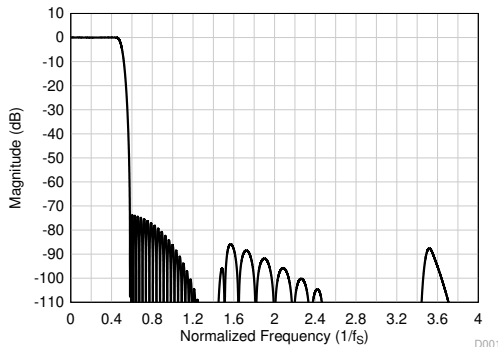
图 6-20. 线性相位抽取滤波器幅度响应
