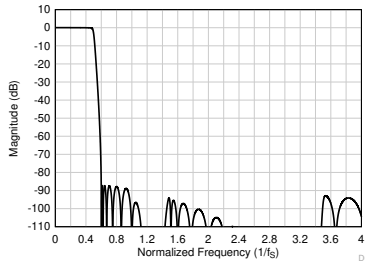
图 6-24. 低延迟抽取滤波器幅度响应
