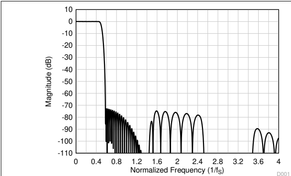
图 6-11. 线性相位抽取滤波器幅度响应
