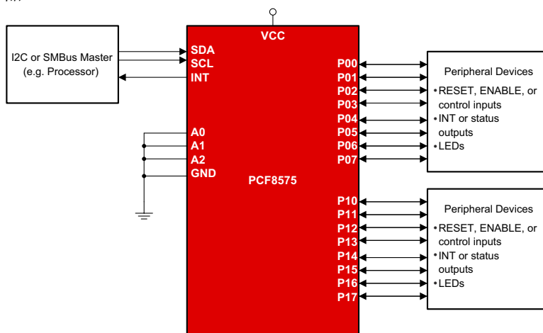
简化原理图
