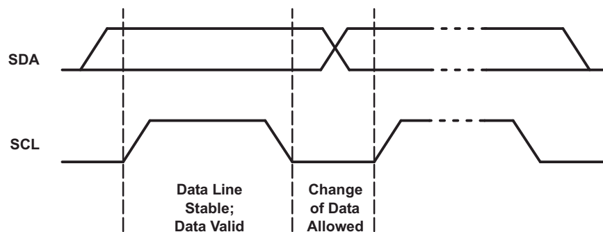
图 8-4. Bit Transfer
