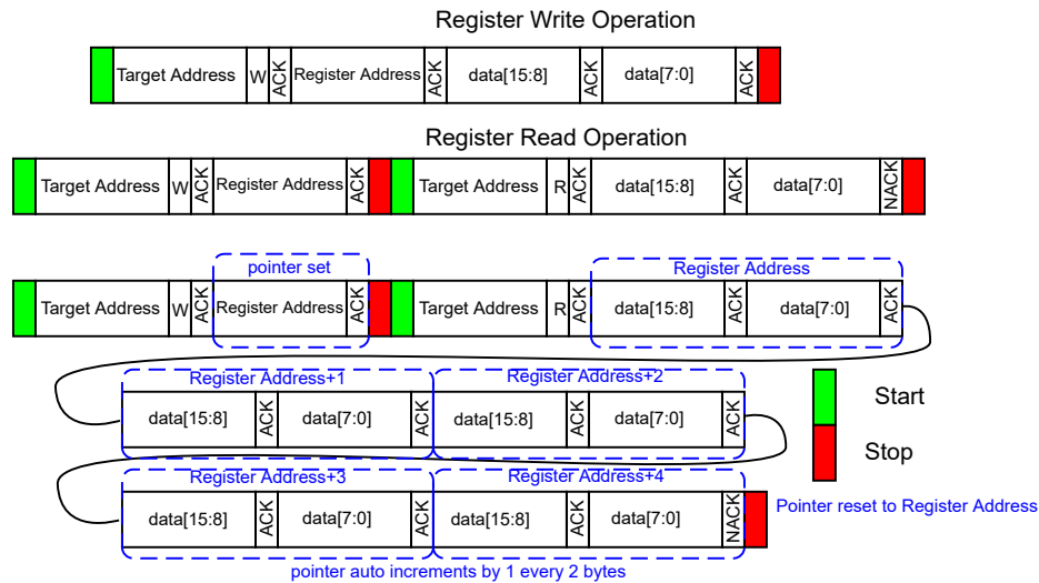
图 6-7. I 2 C 操作
