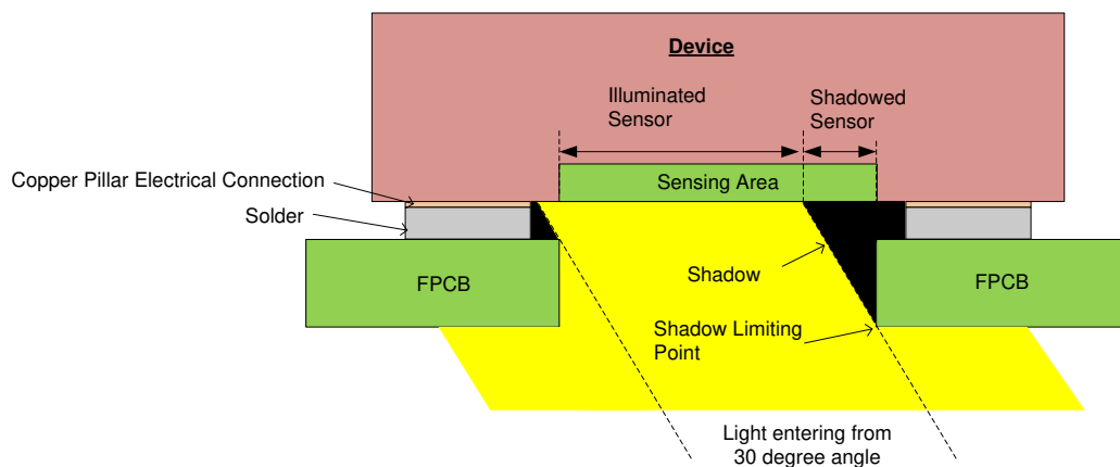
图 8-6. OPT4001-Q1 (焊接到带切口的 FPCB 上, 光从某个角度进入) 横截面图
