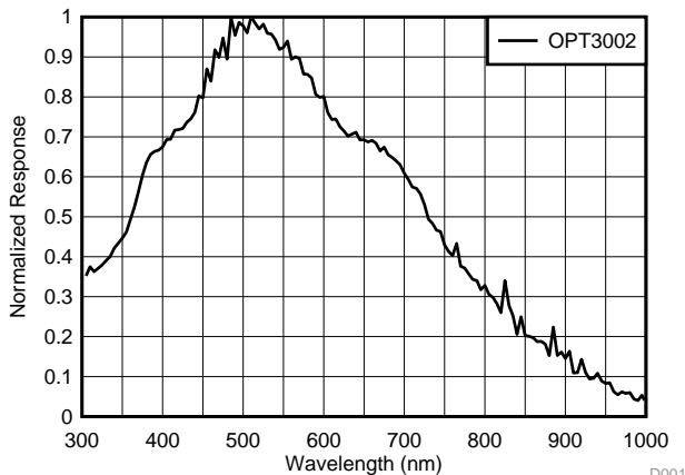
频谱响应
