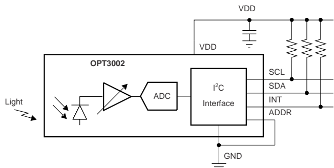
方框图
