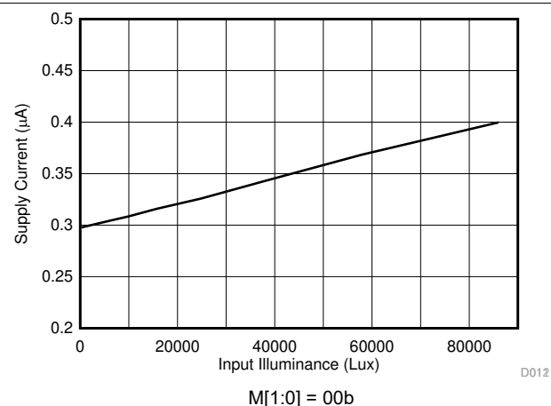
图 5-17. 关断电流与输入照度间的关系
