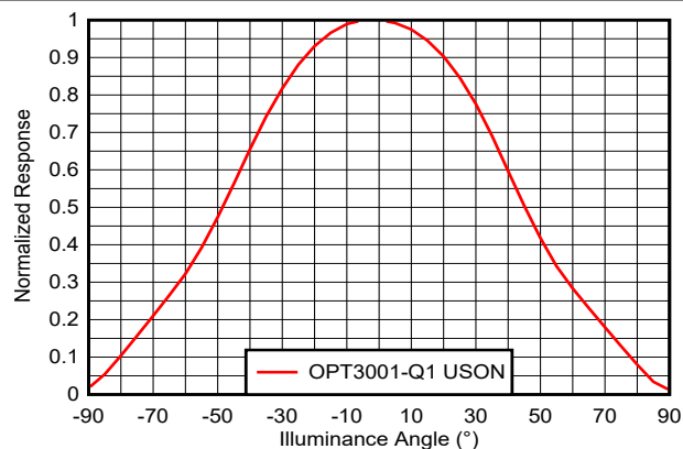
图 5-15. 归一化响应与照明角度间的关系
