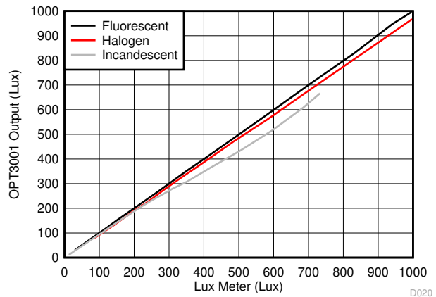
图 8-6. OPT3001-Q1 3 级器件在由荧光灯、卤素灯和白炽灯光源照明的暗窗下的补偿输出
