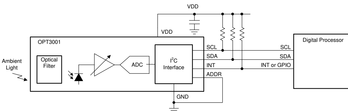
图 8-1. 在产品外壳中和暗窗后测量环境光
