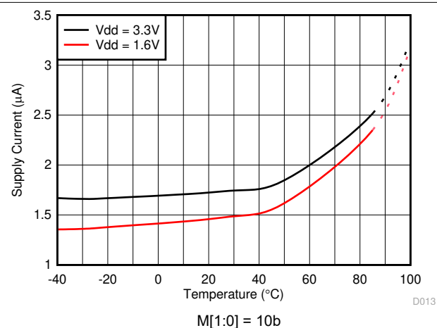
图 5-19. 电源电流与温度间的关系 (3 级)
