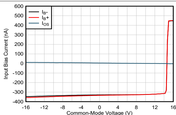
图 5-11. 输入偏置电流和失调电流与共模电压间的关系
