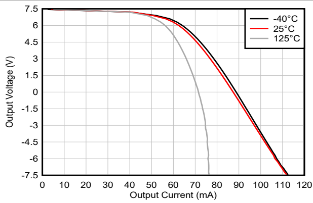
图 5-15. 输出电压摆幅与输出电流 (拉电流) 间的关系
