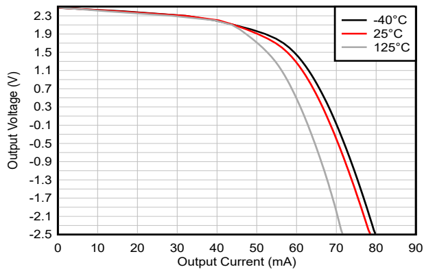
图 5-17. 输出电压摆幅与输出电流 (拉电流) 间的关系
