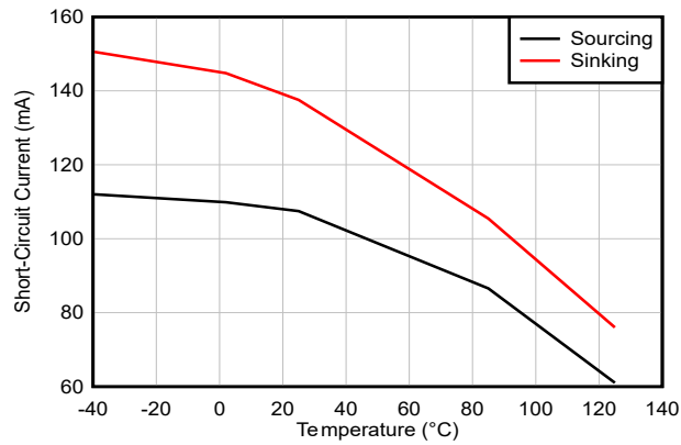
图 5-49. 短路电流与温度间的关系
