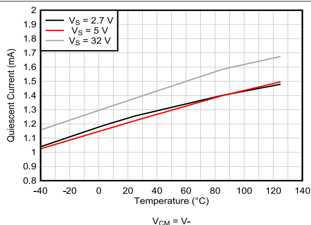
图 5-33. 静态电流与温度间的关系
