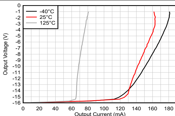
图 5-14. 输出电压摆幅与输出电流 (灌电流) 间的关系
