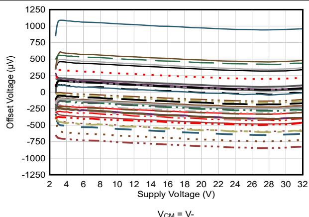
图 5-8. 失调电压与电源间的关系
