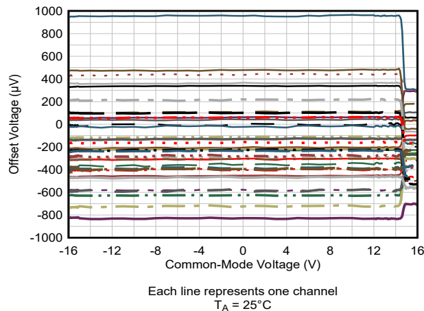
图 5-5. 失调电压与共模电压间的关系
