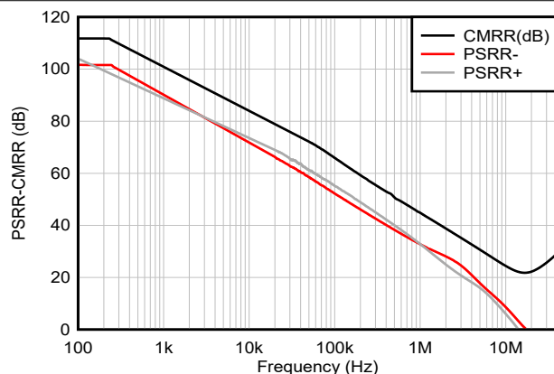
图 5-21. CMRR 和 PSRR 与频率间的关系
