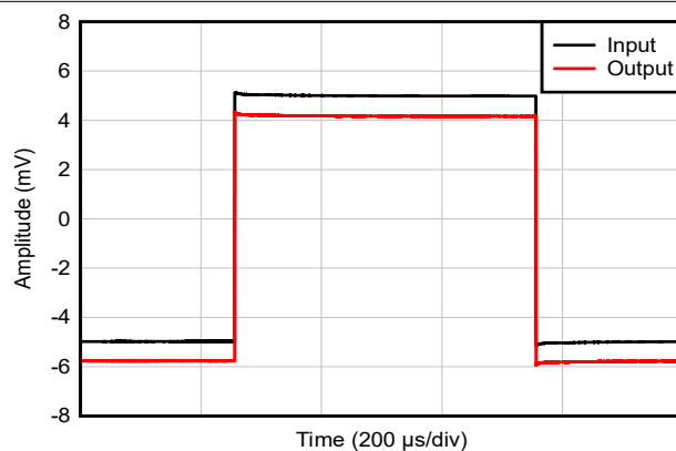
图 5-44. 小信号阶跃响应
