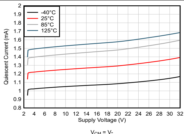
图 5-32. 静态电流与电源电压间的关系
