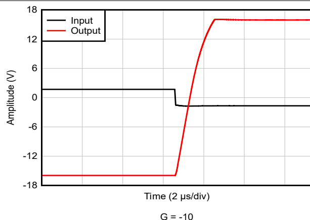
图 5-43. 负过载恢复
