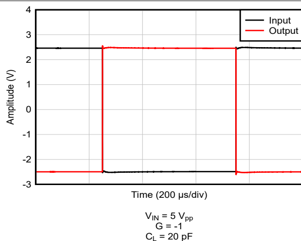
图 5-47. 大信号阶跃响应
