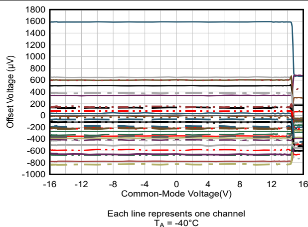
图 5-7. 失调电压与共模电压间的关系
