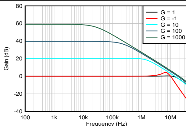
图 5-10. 闭环增益与频率间的关系
