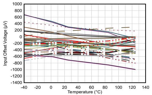
图 5-2. 失调电压漂移分布
