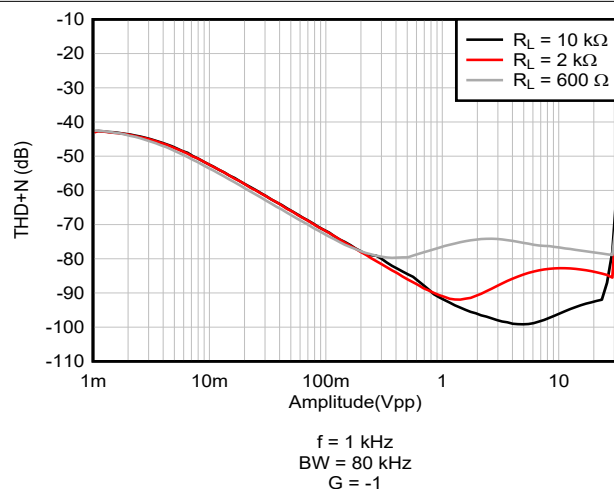
图 5-31. THD+N 与输出幅度间的关系
