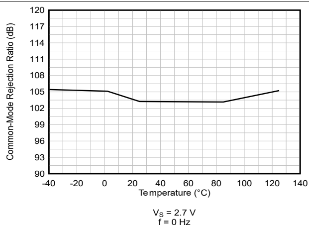
图 5-24. CMRR 与温度间的关系
