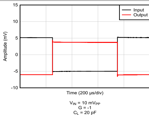
图 5-45. 小信号阶跃响应
