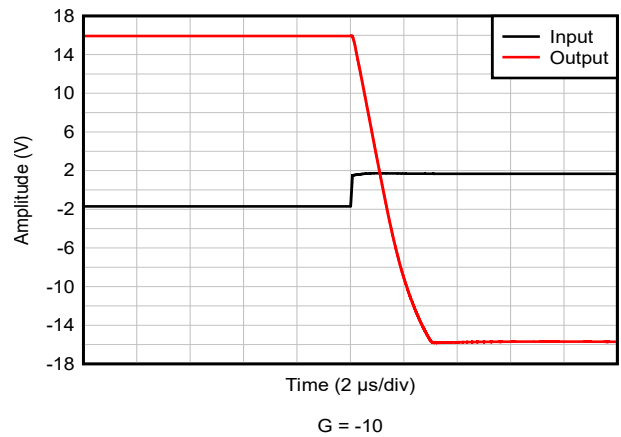
图 5-42. 正过载恢复
