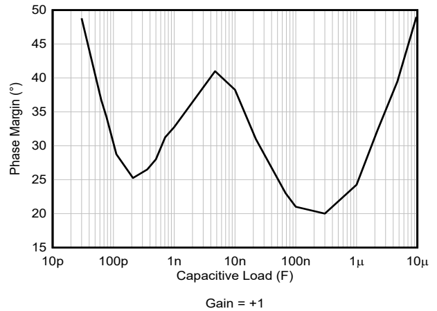
图 5-40. 相位裕度与容性负载间的关系
