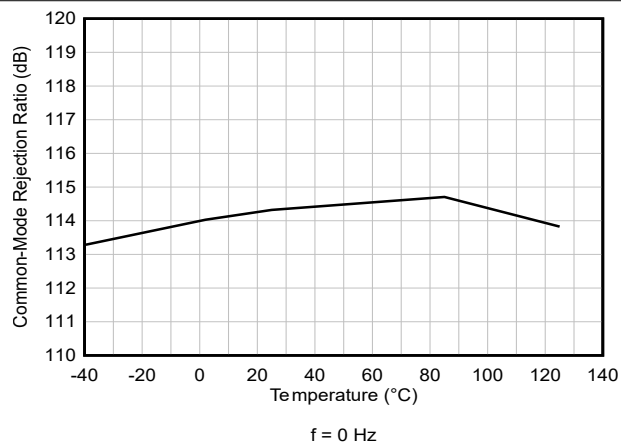
图 5-22. CMRR 与温度间的关系
