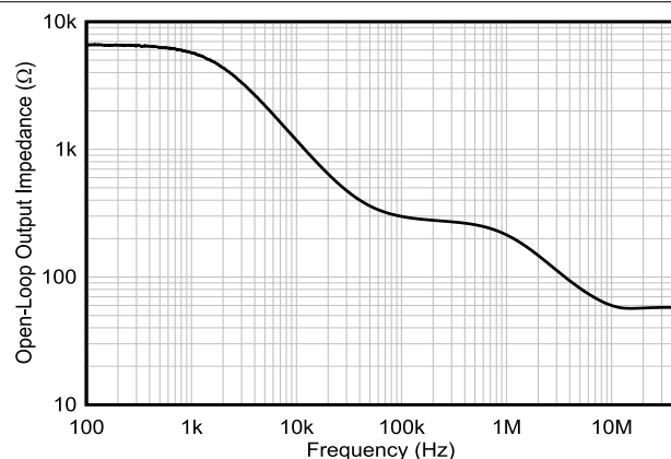
图 5-35. 开环输出阻抗与频率间的关系
