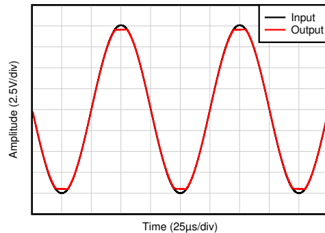
图 6-4. 无相位反转
