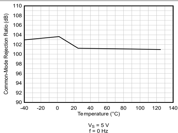
图 5-23. CMRR 与温度间的关系
