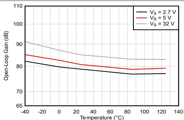
图 5-34. 开环电压增益与温度间的关系 (dB)
