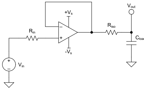
图 6-1. 使用 OPA994-Q1 扩展容性负载驱动
