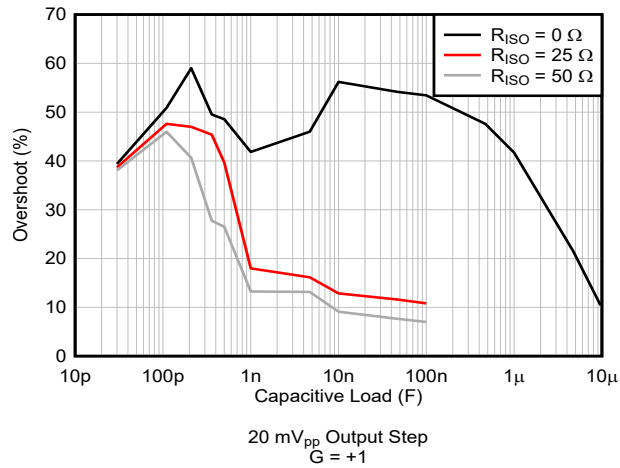
图 5-39. 小信号过冲与容性负载间的关系
