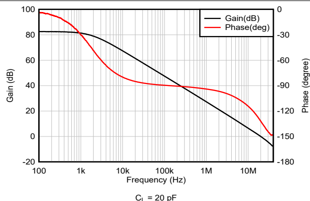
图 5-9. 开环增益和相位与频率间的关系
