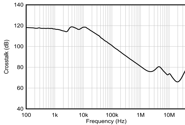
图 5-51. 通道隔离与频率间的关系
