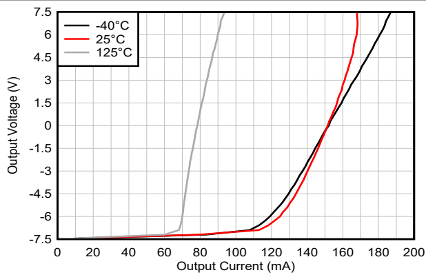
图 5-16. 输出电压摆幅与输出电流 (灌电流) 间的关系
