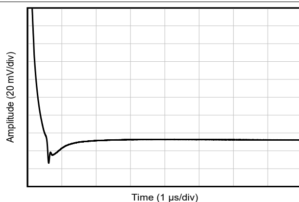
图 5-48. 稳定时间
