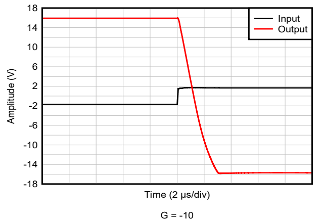
图 5-42. 正过载恢复
