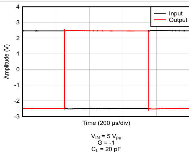
图 5-47. 大信号阶跃响应
