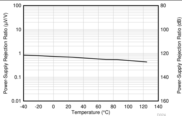
图 5-24. PSRR 与温度间的关系
