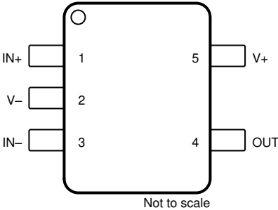
图 4-2. OPA992 DCK 封装 5 引脚 SC70 (顶视图)
