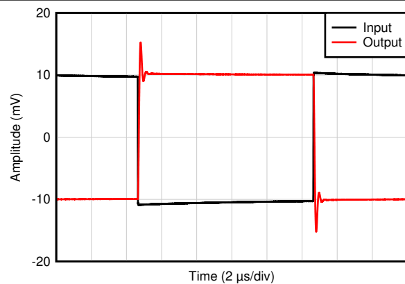
图 5-36. 负过载恢复
