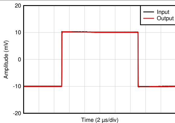
图 5-35. 正过载恢复
