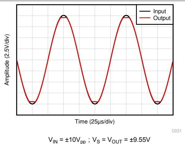
图 5-34. 无相位反转
