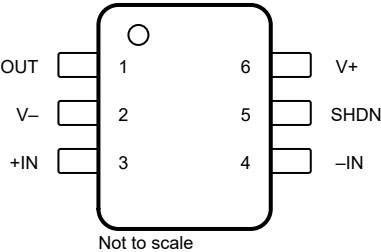
图 4-3. OPA992S DBV 封装 6 引脚 SOT-23 (顶视图)
