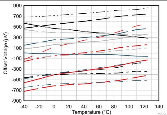
V_{CM} = V_+
