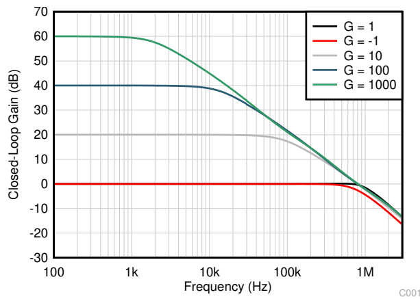
图 6-11. 闭环增益与频率间的关系
