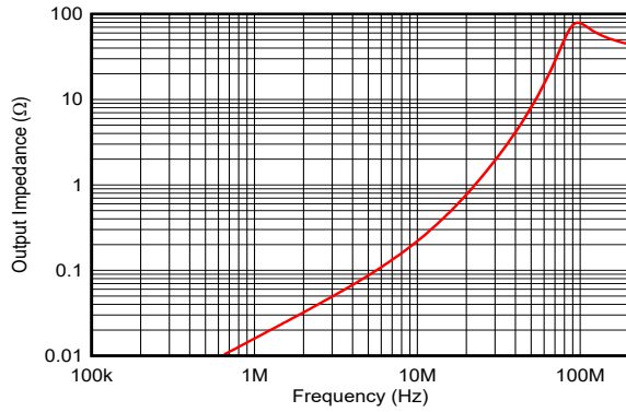
图 5-7. 闭环输出阻抗
