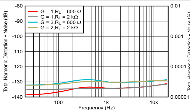
图 5-33. THD+N 与频率间的关系
