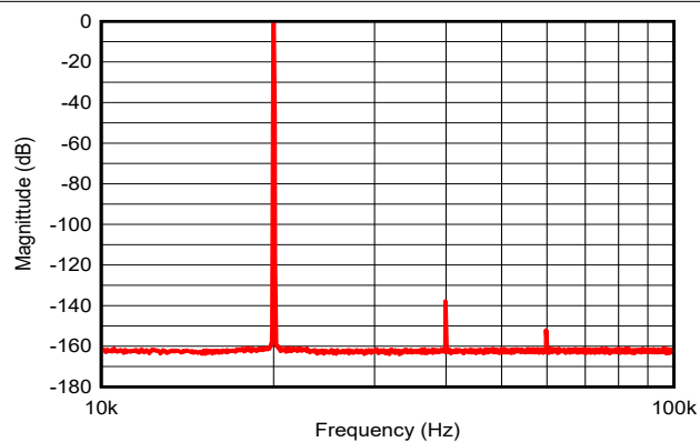
图 5-44. 20kHz 输出频谱
