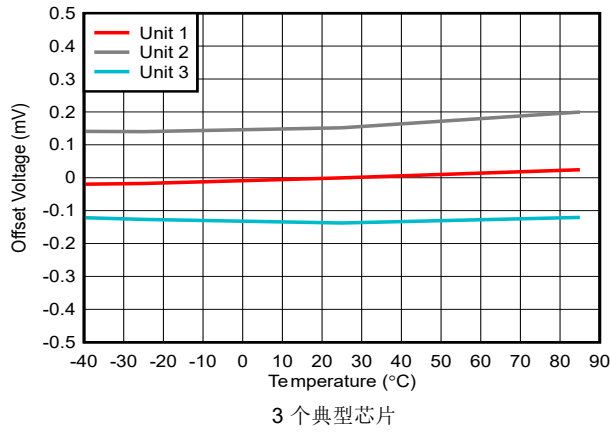
图 5-25. 输入失调电压与环境温度间的关系
