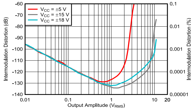
图 5-37. 互调失真与振幅间的关系
