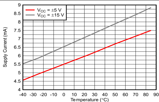
图 5-32. 电源电流与环境温度间的关系
