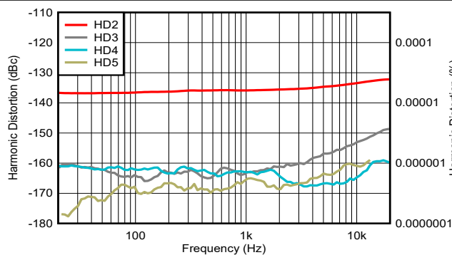
图 5-39. 谐波失真与频率间的关系
