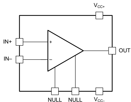
图 6-1. OPA891 : 单通道
