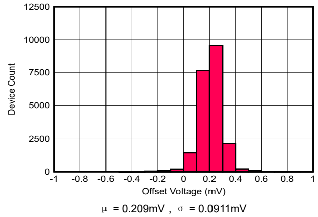
图 5-26. 失调电压分布
