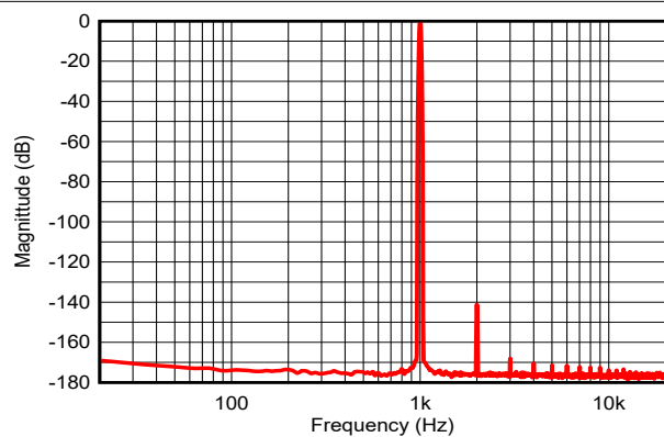
图 5-43. 1kHz 输出频谱
