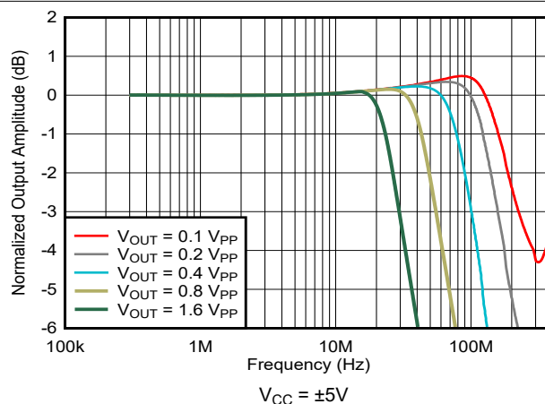
图 5-8. 大信号频率响应
