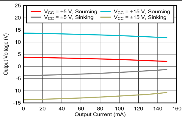
图 5-31. 输出摆幅与负载电流间的关系
