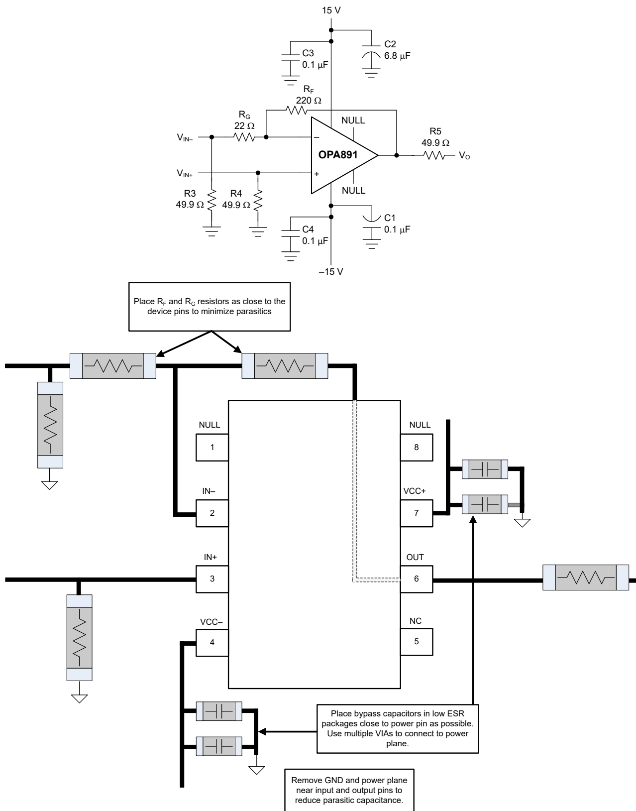
图 7-11. 布局建议
