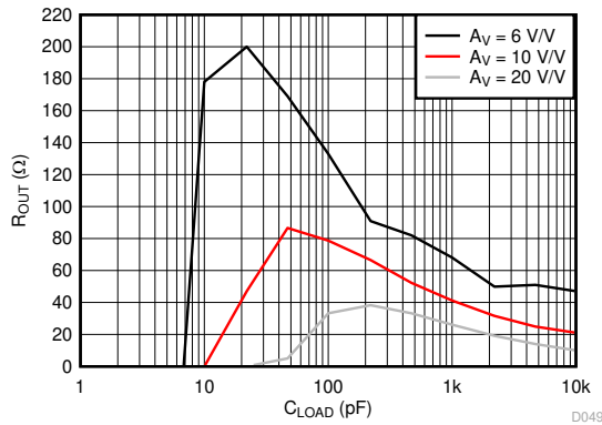
图 6-49. Output Resistor vs C_{\text{LOAD}}
