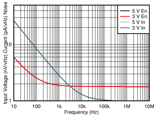
图 6-39. Input Spot Noise Density
