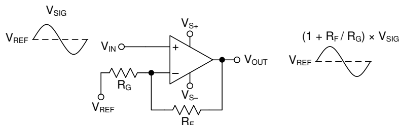
图 7-1. 同相放大器
