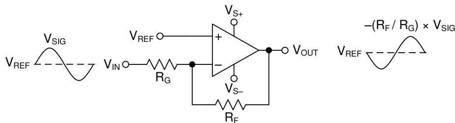
图 7-2. 反相放大器
