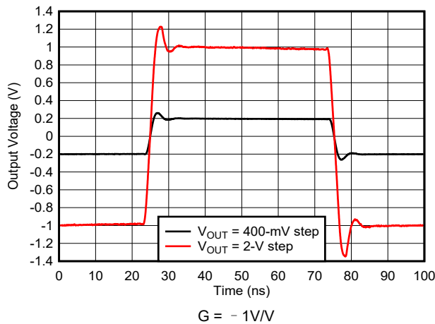
图 6-11. 反相大信号脉冲响应
