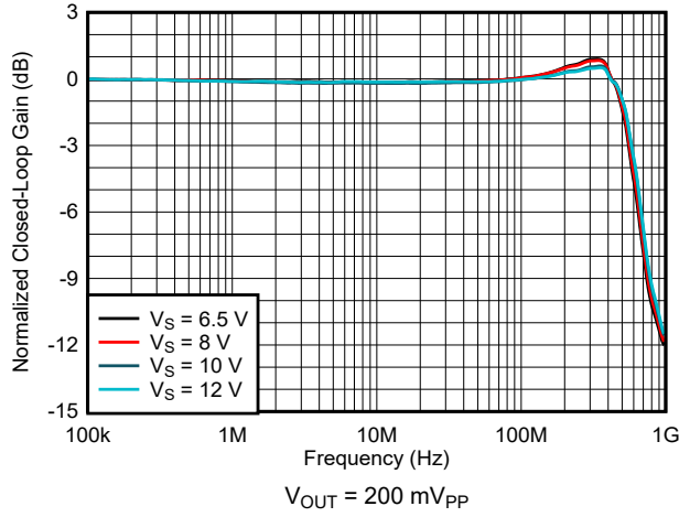
图 6-7. 电源上的同相小信号频率响应
