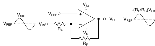
图 8-4. Inverting Amplifier
