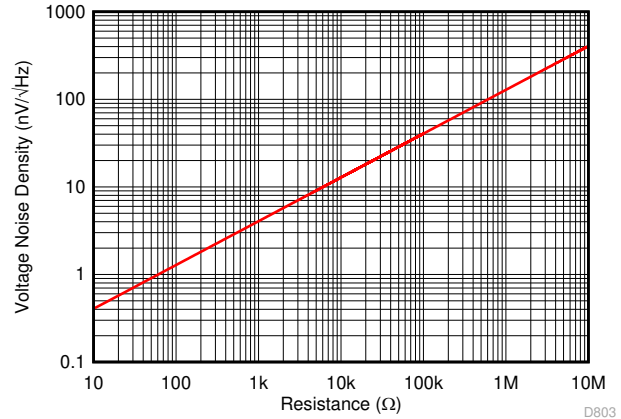
图 8-9. Thermal Noise Density vs Resistance
