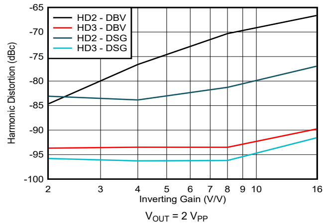
图 5-12. 10MHz 谐波失真与反相增益间的关系
