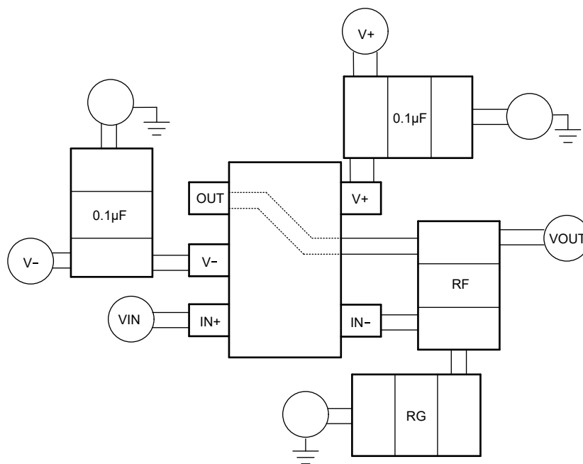
图 7-10. SOT23-5 封装同相配置的电路板布局布线
