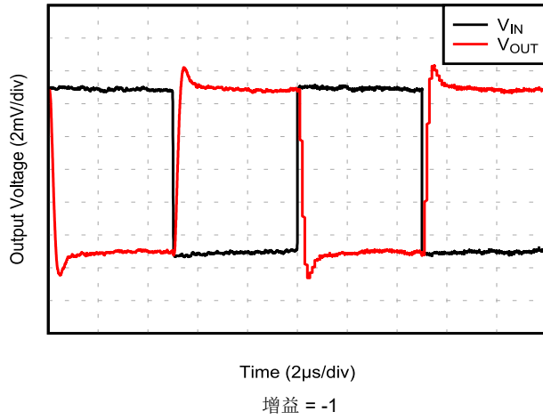
图 5-33. 小信号阶跃响应
