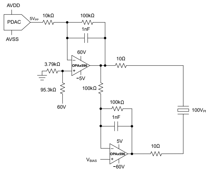
图 7-1. 具有桥式连接负载的 100\text{V}_{\text{PP}} 压电式驱动器
