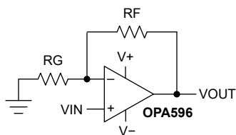
图 7-9. 同相配置的原理图表示
