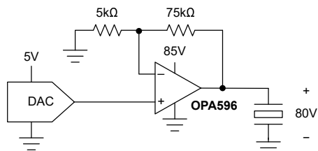
图 7-4. 80V 单电源压电式驱动器
