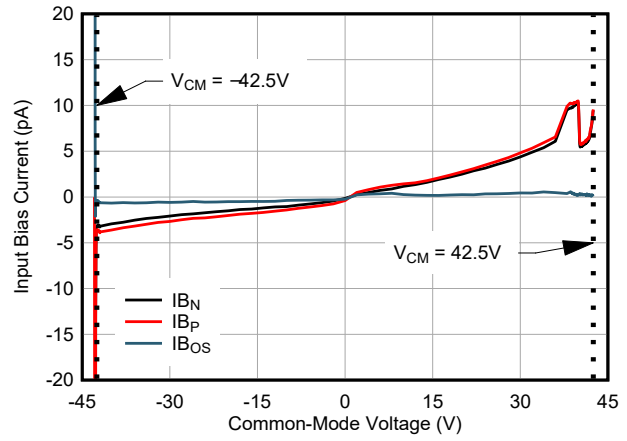
图 5-10. 输入偏置与共模电压间的关系
