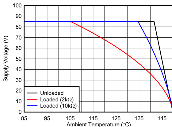
图 7-8. OPA596 (SOT23-5) 热安全工作区
