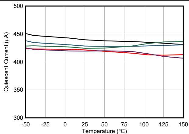
图 5-38. 静态电流与温度间的关系
