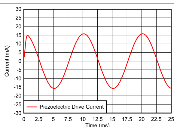
图 7-3. 压电式驱动器输出电流
