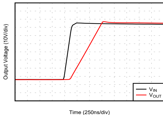
大信号阶跃响应
