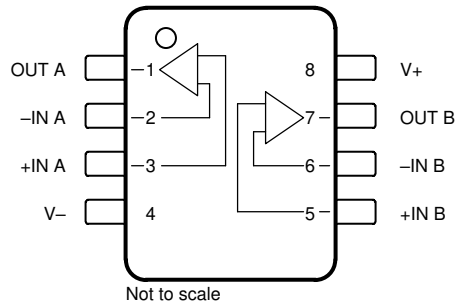
图 4-2. OPA2596 D 预发布封装，8 引脚 SOIC 和 DGK 预发布封装，8 引脚 VSSOP (顶视图)
