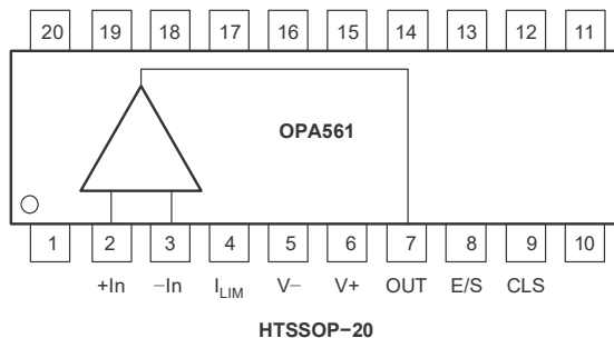
引脚排列图
