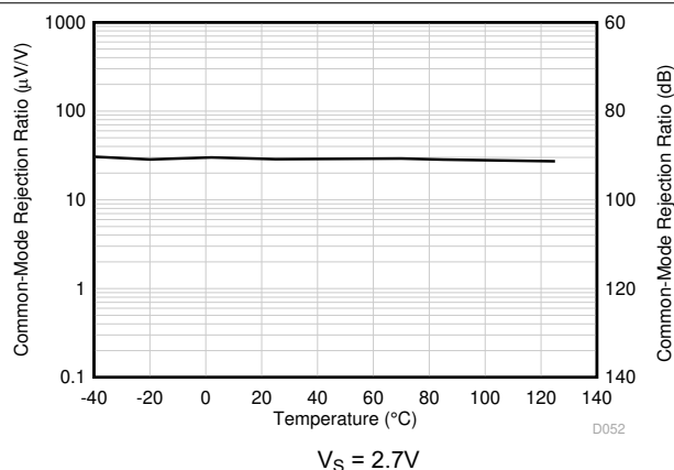
图 5-23. CMRR vs Temperature
