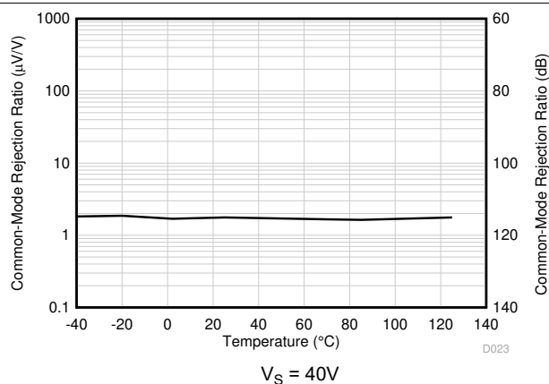
图 5-21. CMRR vs Temperature
