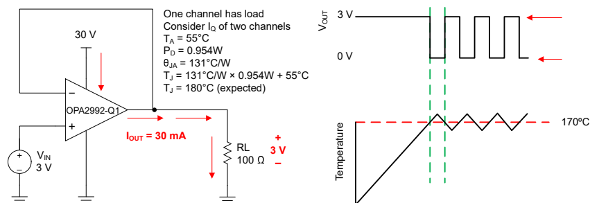
图 6-4. Thermal Protection
