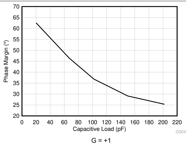
图 5-33. Phase Margin vs Capacitive Load
