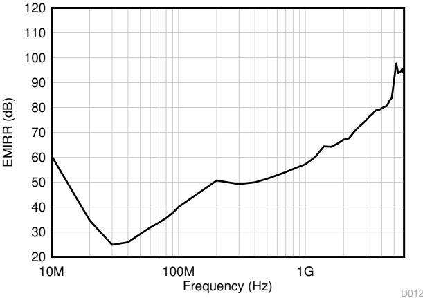
图 6-3. EMIRR Testing
