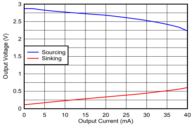
图 7-37. Output Voltage vs Load Current
