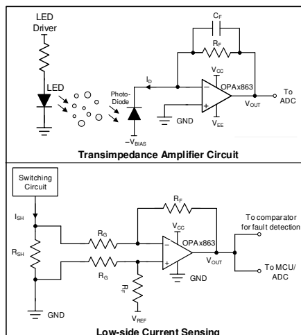
使用 OPAx863 的应用电路
