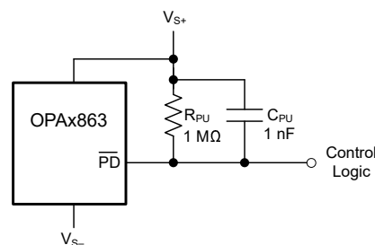
图 8-2. Power Down Control
