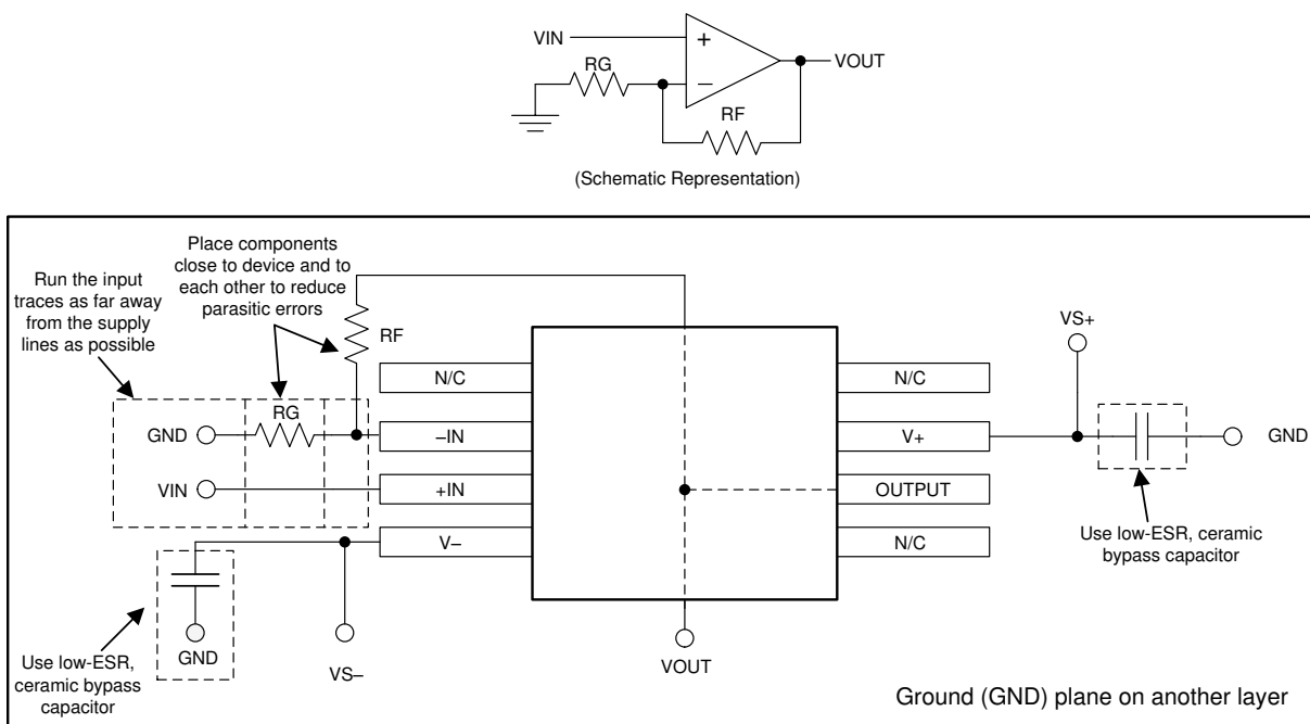
图 10-1. Layout Example
