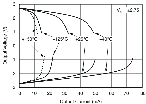
图 6-14. Output Voltage vs Output Current
