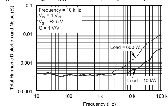
图 19. THD+N 与频率间的关系
