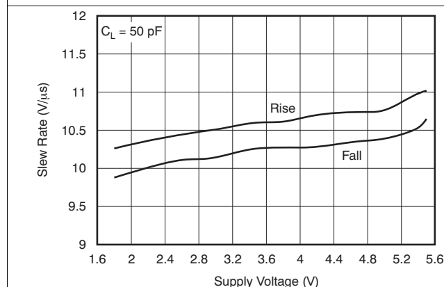
图 21. 压摆率与电源电压间的关系
