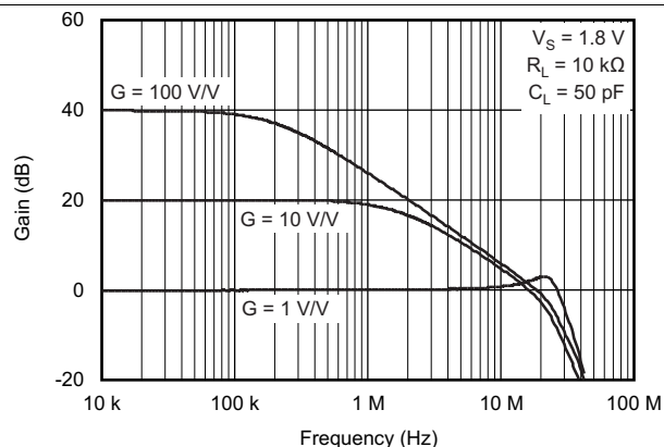
图 11. 闭环增益与频率间的关系
