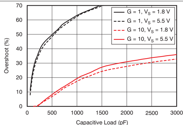
图 16. 小信号过冲 与负载电容间的关系
