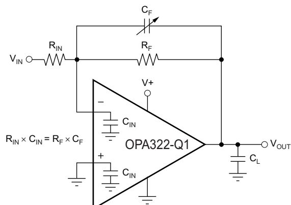
图 28. 反馈电容器提高动态性能
