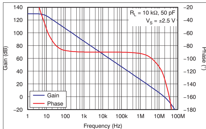
图 1. 开环增益和相位与频率间的关系
