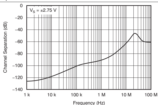
图 20. 通道分离与频率间的关系 (双通道)
