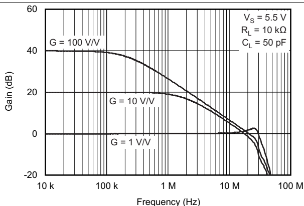
图 12. 闭环增益与频率间的关系
