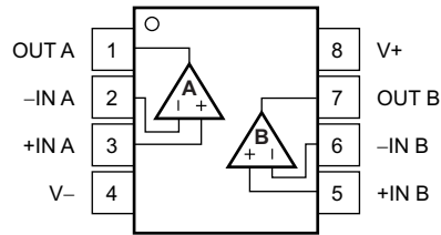
引脚功能：OPA2322-Q1
