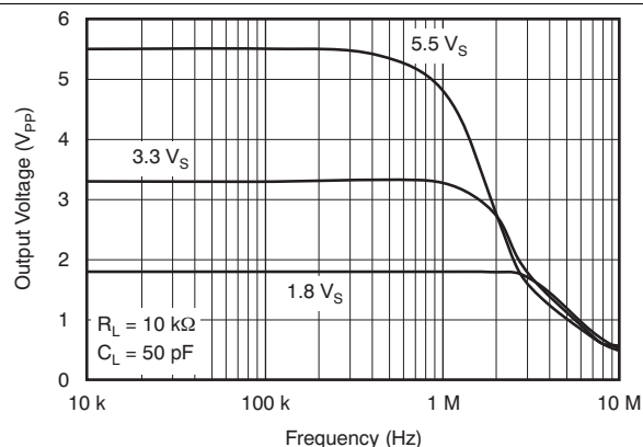
图 13. 最大输出电压与频率间的关系
