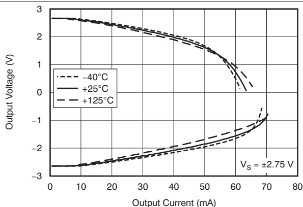
图 14. 输出电压摆幅与输出电流间的关系
