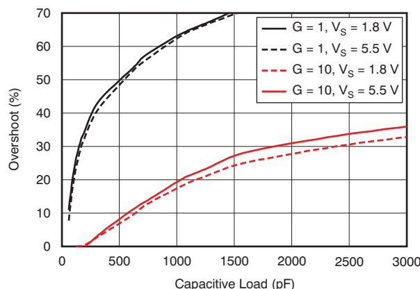
图 29. 小信号过冲与容性负载间的关系 (100mV pp 输出阶跃)
