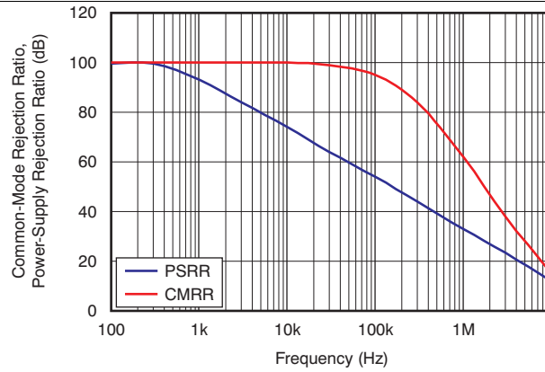
图 25. CMRR 和 PSRR 与频率间的关系
