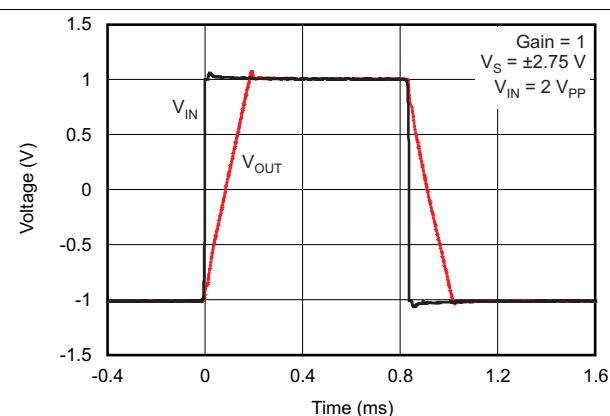
图 24. 大信号阶跃响应与时间间的关系
