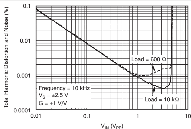
图 17. THD+N 与幅度间的关系
