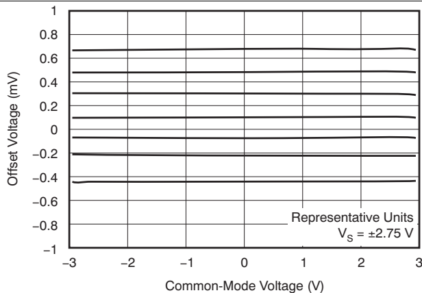
图 8. 失调电压与共模电压间的关系
