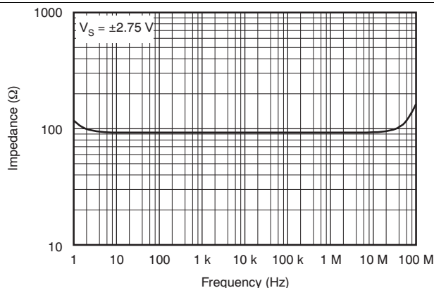
图 15. 开环输出阻抗 与频率间的关系
