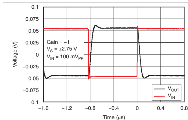
图 23. 小信号阶跃响应
