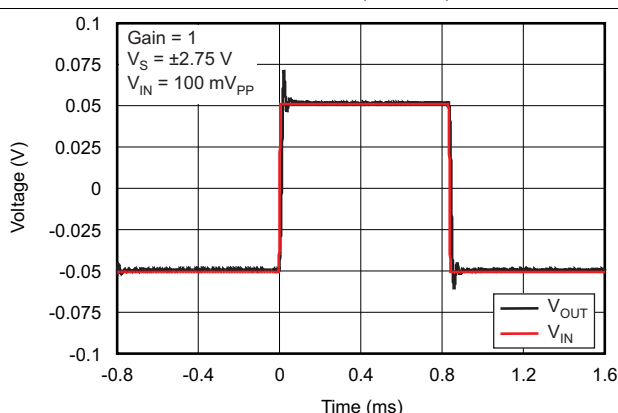
图 22. 小信号阶跃响应
