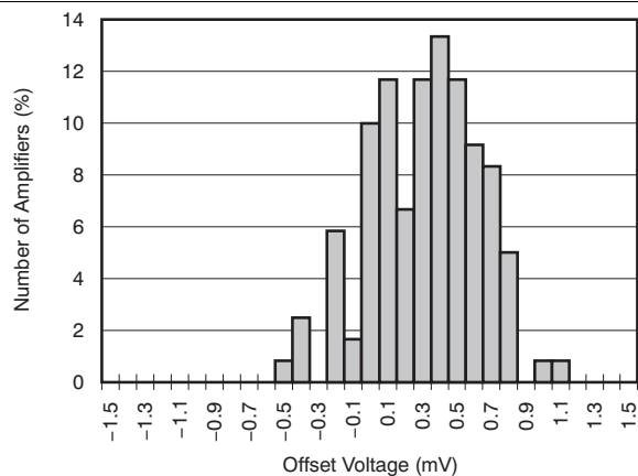
图 7. 失调电压产生直方图
