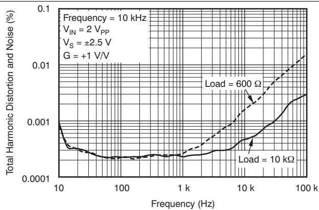
图 18. THD+N 与频率间的关系
