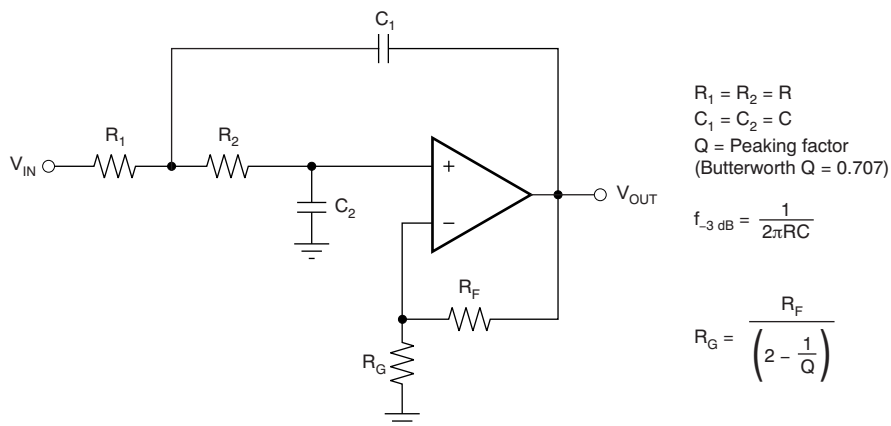
图 40. 两极低通 Sallen-Key 滤波器
