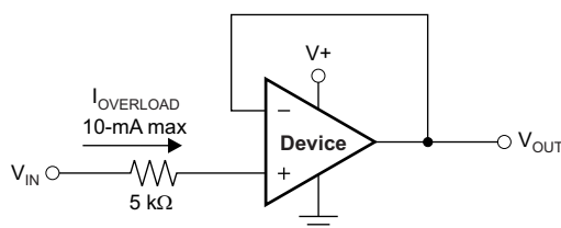
图 37. 输入电流保护
