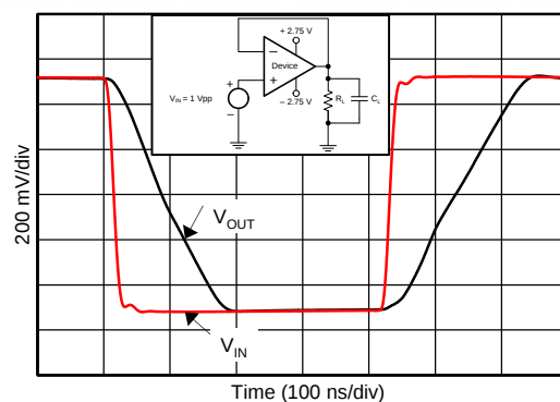
图 28. 负过载恢复
