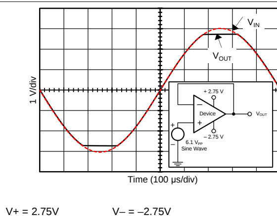
图 26. 无相位反转
