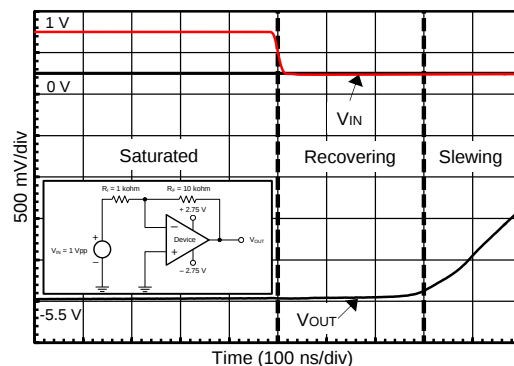
图 26. 无相位反转
