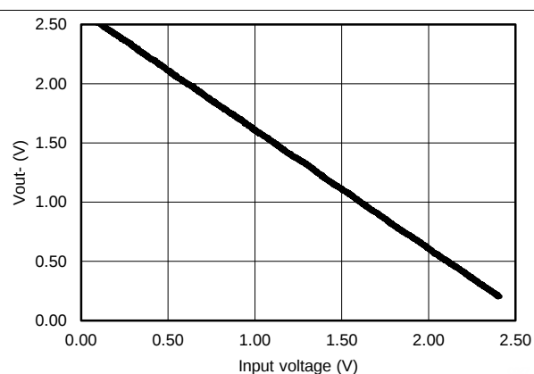
图 39. V_{OUT-} 与输入电压间的关系
