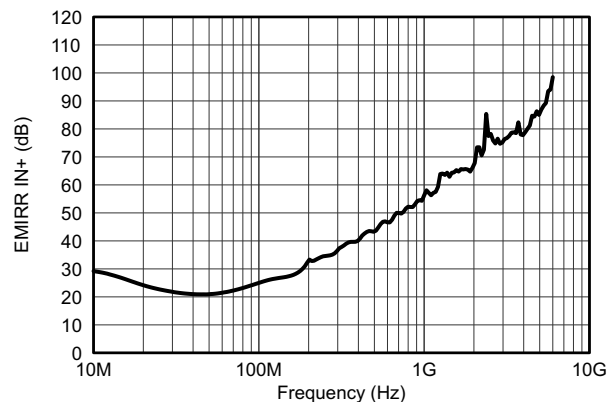
EMIRR 与频率间的关系
