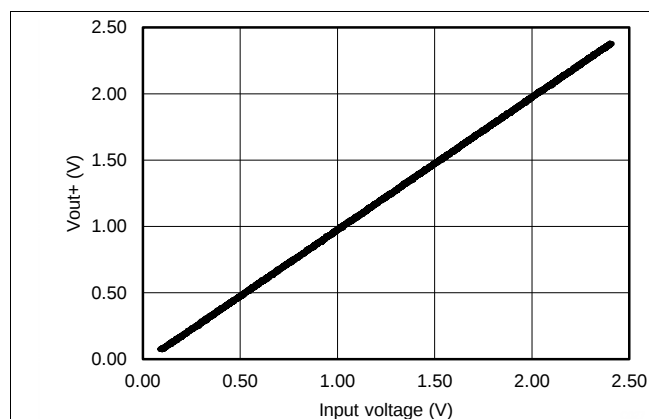
图 38. V_{OUT+} 与输入电压间的关系
