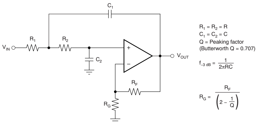
图 35. 两极点低通 Sallen-Key 滤波器
