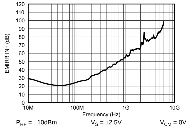
图 32. 以同相输入为参考的电磁干扰抑制比 (EMIRR IN+) 与频率间的关系
