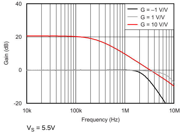
图 19. 闭环增益与频率间的关系
