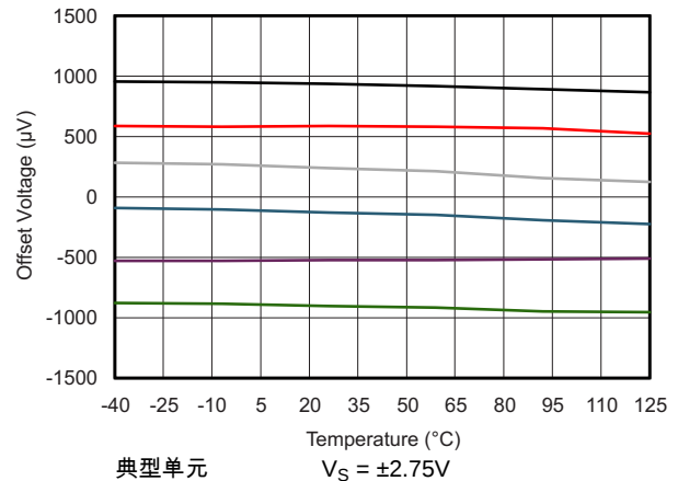
图 8. 失调电压与温度间的关系
