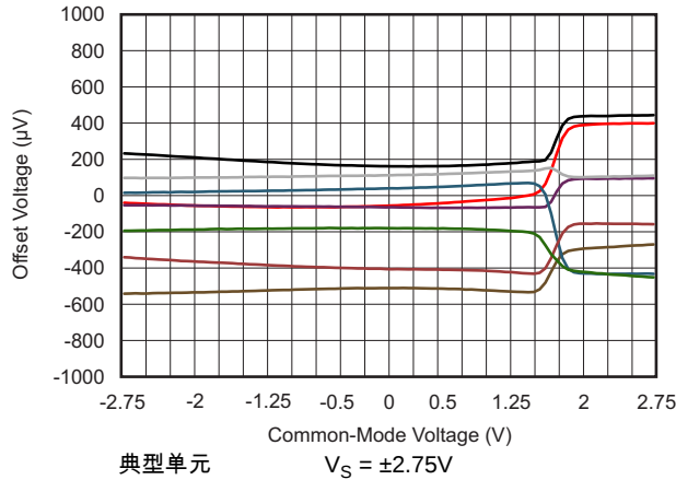
图 7. 失调电压与共模电压间的关系
