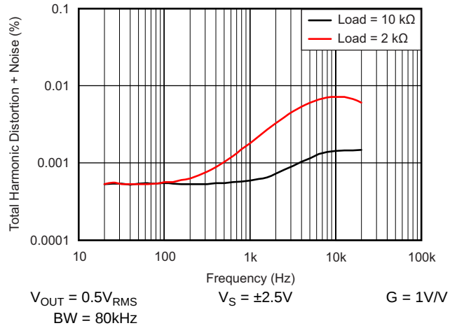
图 31. THD+N 与频率间的关系
