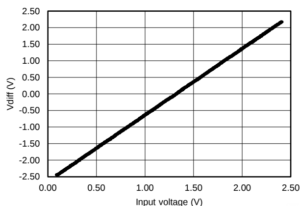
图 40. V_{DIFF} 与输入电压间的关系
