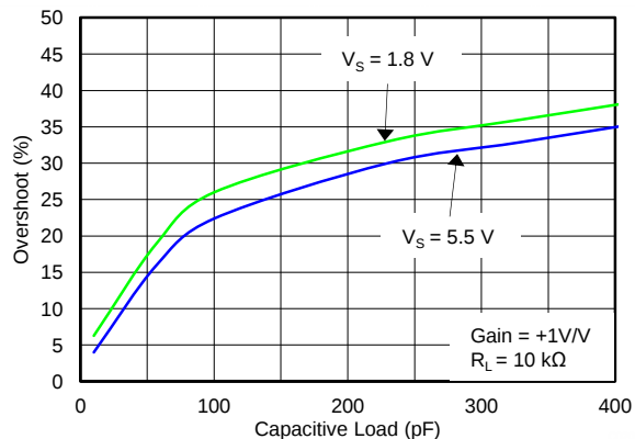
Figure 20. 小信号过冲与负载电容间的关系
