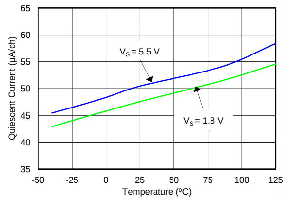
Figure 4. 静态电流与温度间的关系
