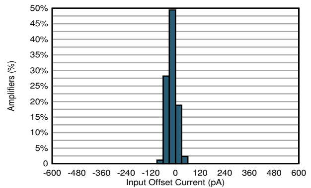
图 7-4. 输入失调电流产生分布
