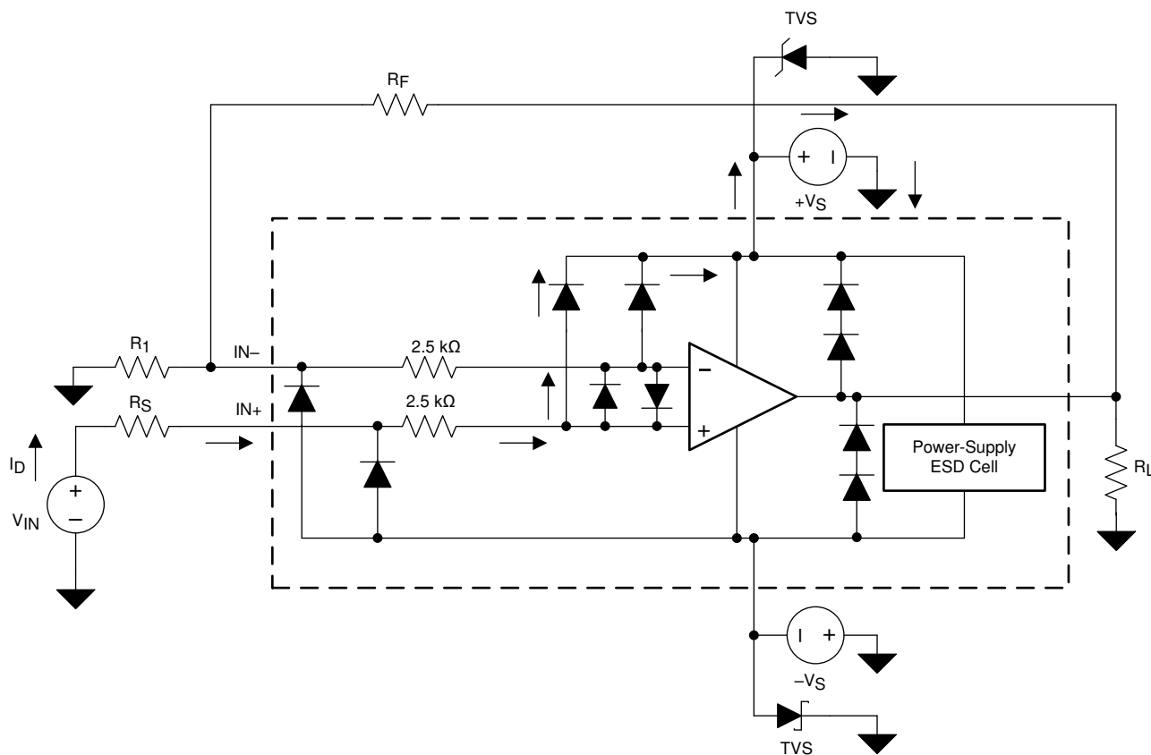
图 7-1. 与典型电路应用相关的等效内部 ESD 电路
