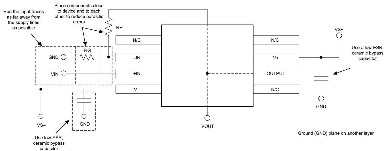
图 7-7. 同相配置的运算放大器电路板布局
