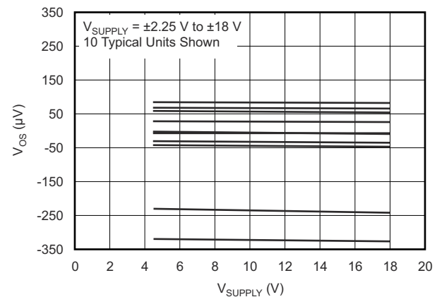
图 5-6. 失调电压与电源间的关系
