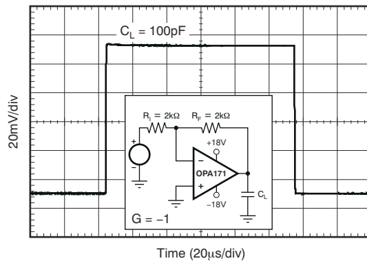
图 5-29. 小信号阶跃响应 (100mV)
