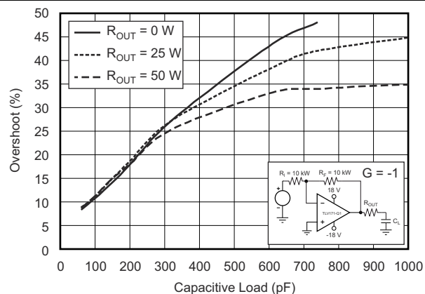
图 5-24. 小信号过冲与容性负载间的关系 (100mV 输出阶跃)
