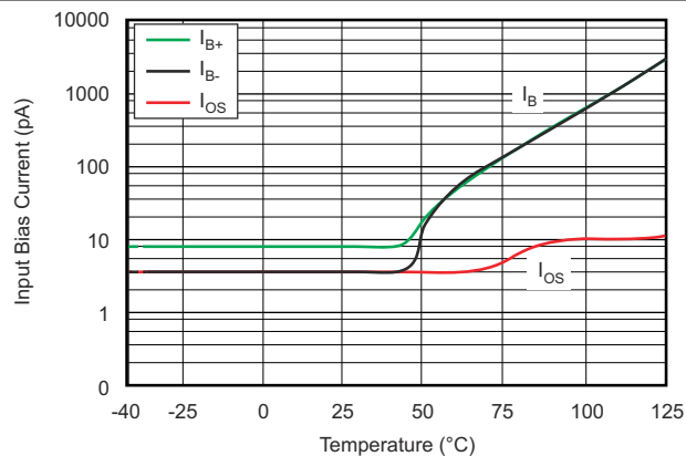
图 5-8. 输入偏置电流与温度间的关系
