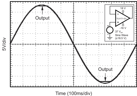
图 6-1. 无相位反转
