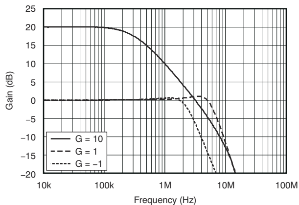
图 5-20. 闭环增益与频率间的关系
