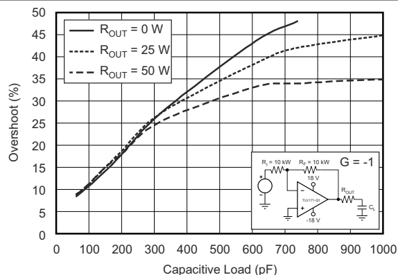
图 7-5. 小信号过冲与容性负载间的关系 ( 100mV 输出阶跃 )
