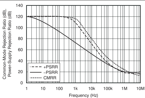
图 5-10. CMRR 和 PSRR 与频率间的关系 (以输入为基准)
