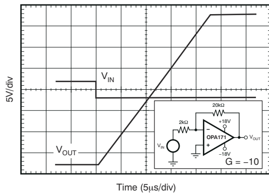
图 5-27. 负过载恢复
