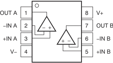
图 4-4. OPA2171 D、DCU 和 DCK 封装：8 引脚 SO 和 VSSOP（顶视图）
