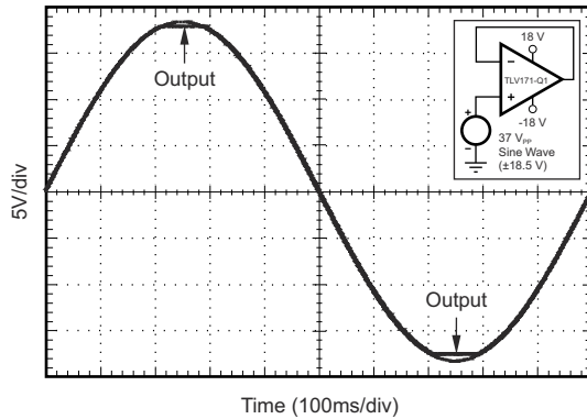
图 5-25. 无相位反转
