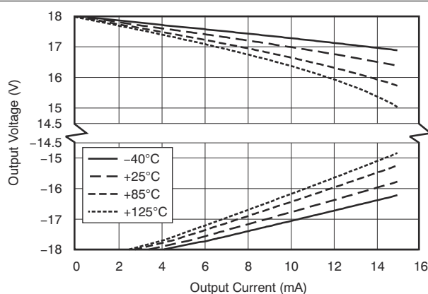
图 5-9. 输出电压摆幅与输出电流间的关系 (最大电源电压)
