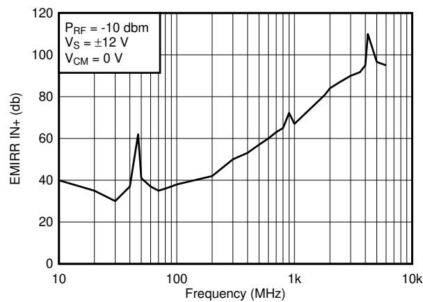
图 7-6. OPA2140 EMIRR
