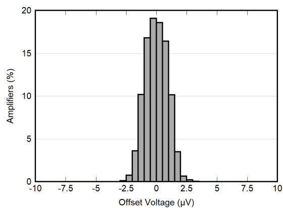
图 6-1. 失调电压分布图
