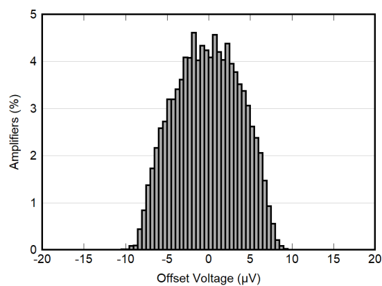
图 6-2. 失调电压分布图
