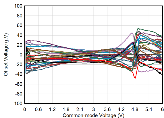
图 6-2. 失调电压分布图
