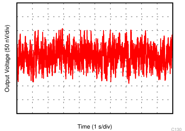
图 6-14. 0.1-Hz to 10-Hz Noise
