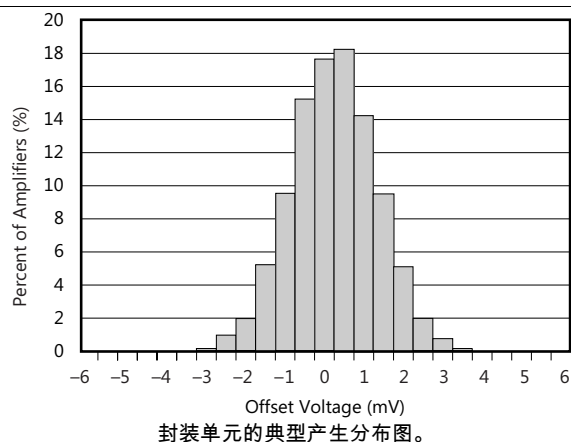
Figure 11. 失调电压分布
