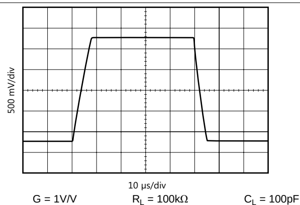
Figure 16. 大信号阶跃响应
