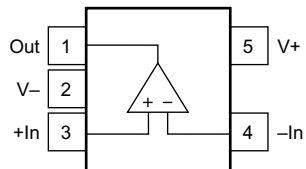
DBV 封装 : OPA348-Q1 5 引脚 SOT-23 俯视图
