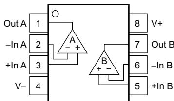
引脚功能 : OPA2348-Q1
