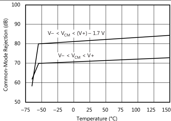
Figure 7. 共模抑制与温度间的关系
