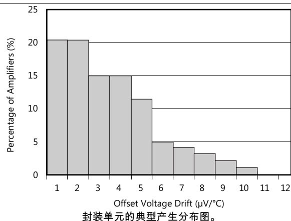
Figure 12. 失调电压漂移幅度产生分布图
