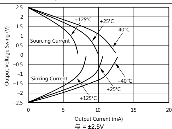
Figure 6. 输出电压摆幅与输出电流间的关系 与 \pm 2.5\text{V}
