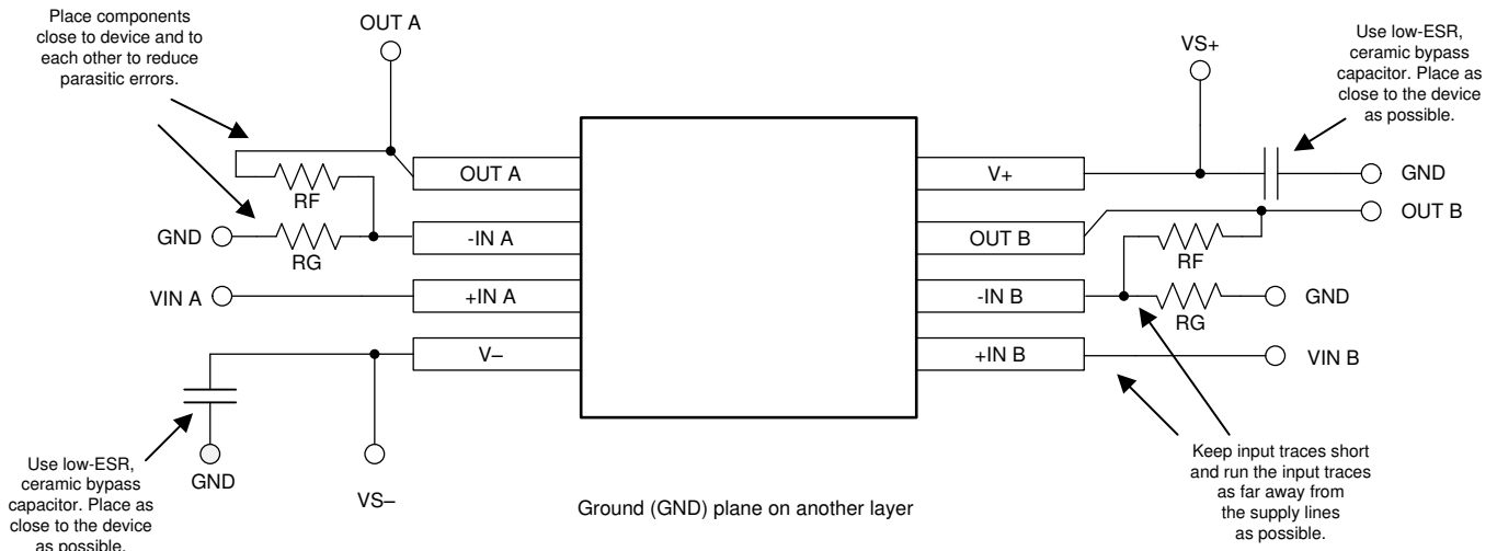
图 57. Layout Example
