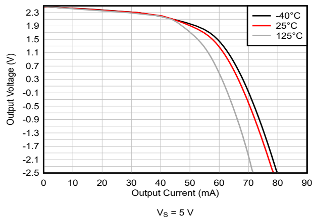
图 5-17. 输出电压摆幅与输出电流 (拉电流) 间的关系
