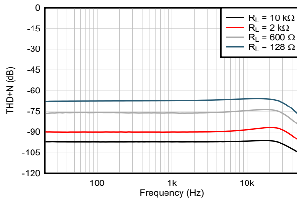
图 5-29. THD+N 比与频率间的关系 G = -1 V_{OUT} = 3 V_{RMS} BW = 80\text{ kHz}
