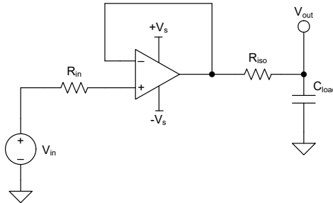
图 6-1. 使用 OPA994 扩展容性负载驱动
