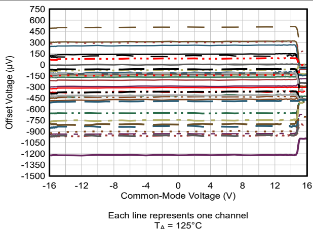
图 5-6. 失调电压与共模电压间的关系
