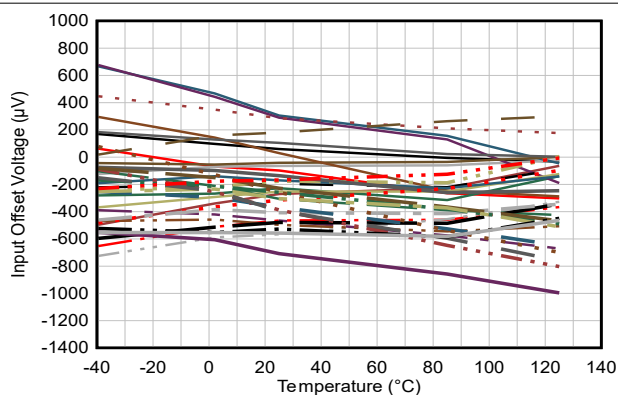
图 5-2. 失调电压漂移分布
