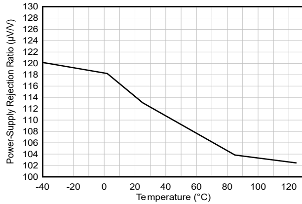
图 5-25. PSRR 与温度间的关系 f = 0\text{ Hz}
