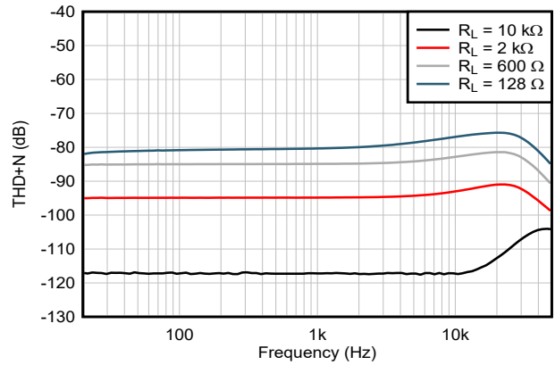
图 5-28. THD+N 比与频率间的关系 G = +1 V_{OUT} = 3 V_{RMS} BW = 80\text{ kHz}
