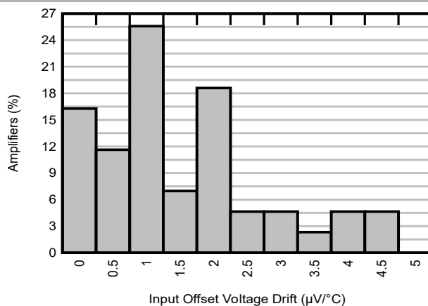
图 5-2. 失调电压漂移分布
