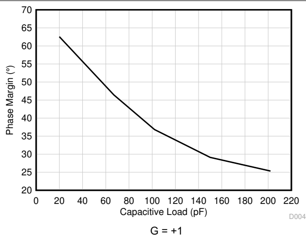
图 5-33. Phase Margin vs Capacitive Load
