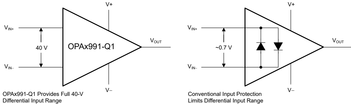
图 6-1. OPA x 991-Q1 输入保护不限制差分输入能力
