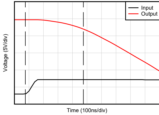
G = -10 图 5-31. 正过载恢复
