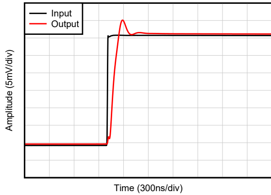
C_L = 20\text{pF} , G = 1 , 20mV 阶跃响应 图 5-33. 小信号阶跃响应, 上升
