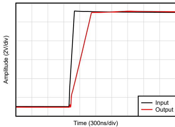
C_L = 20\text{pF} , G = 1 图 5-35. 大信号阶跃响应 (上升)
