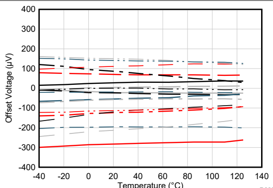
V_{CM} = V_-
