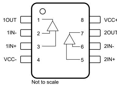
图 4-2. OPA2891 : D 封装 8 引脚 SOIC 或 DGN 封装 8 引脚 HVSSOP ( 顶视图 )
