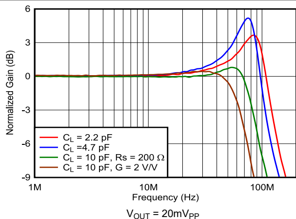
图 6-3. 频率响应与电容负载间的关系
