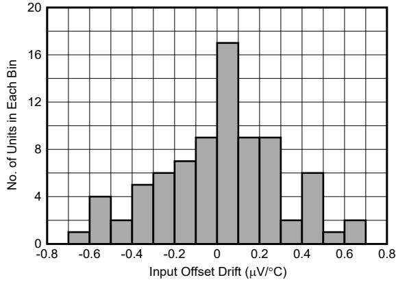
图 6-19. 输入失调电压漂移分布
