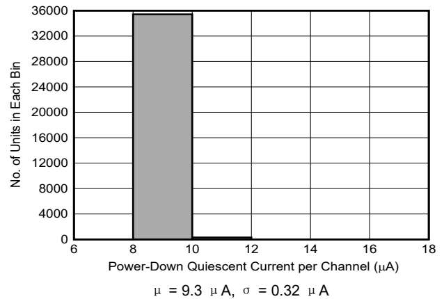
图 6-24. 关断静态电流分布
