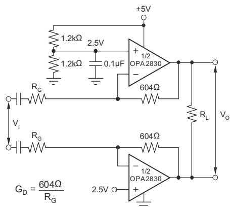
图 7-2. 5V 差分配置测试电路
