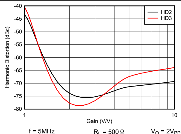
图 6-31. 谐波失真与同相增益间的关系
