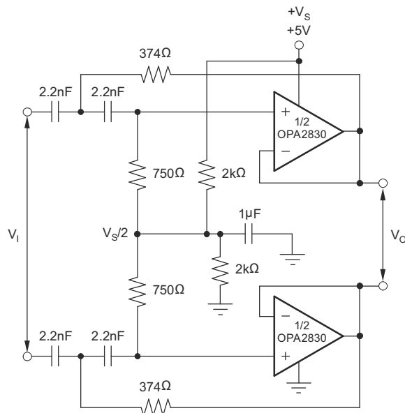
图 8-12. 138kHz、二阶高通滤波器
