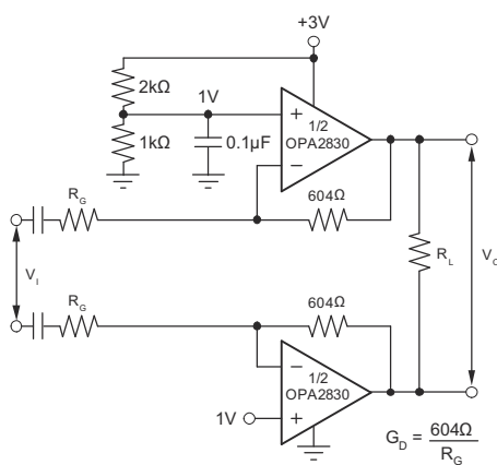
图 7-3. 3V 差分配置测试电路
