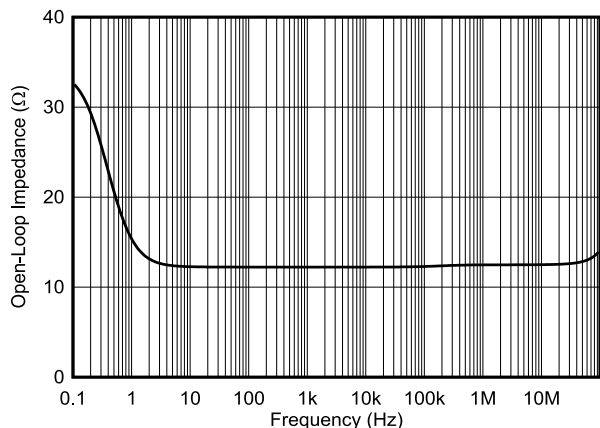
图 6-27. 开环输出阻抗与频率间的关系
