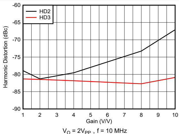
图 7-35. 谐波失真与同相增益间的关系
