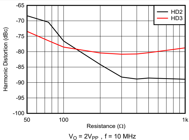
图 7-34. 谐波失真与负载电阻间的关系
