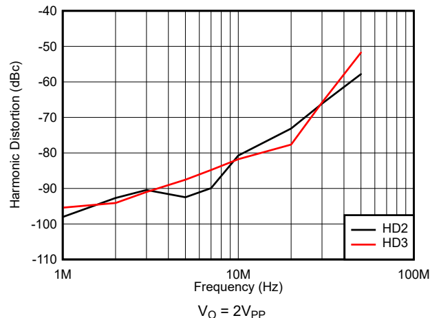
图 7-32. 谐波失真与频率间的关系
