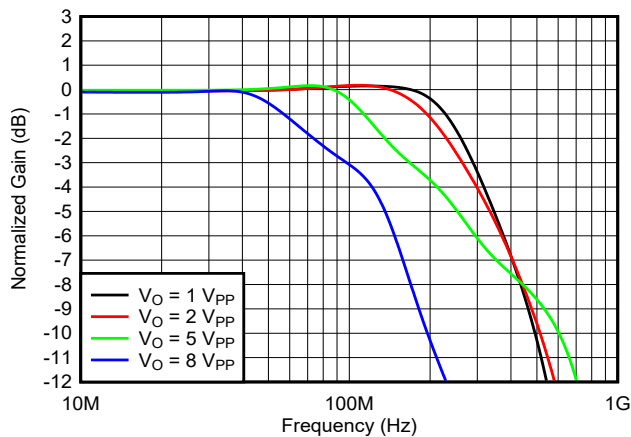
图 7-31. 大信号频率响应
