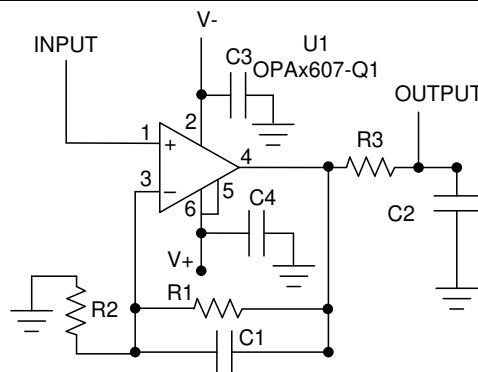
图 11-2. Layout Example Schematic
